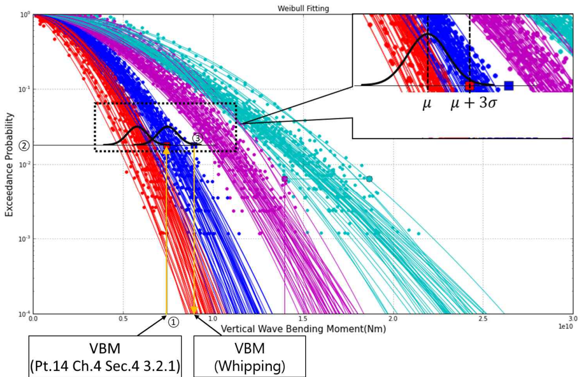
그림 4.3 누적확률분포자료의 Weibull 피팅 (2022)
