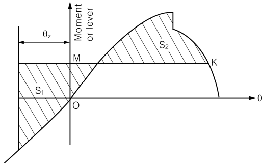
그림 5.1 정복원력
