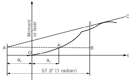
그림 5.2 동복원력
