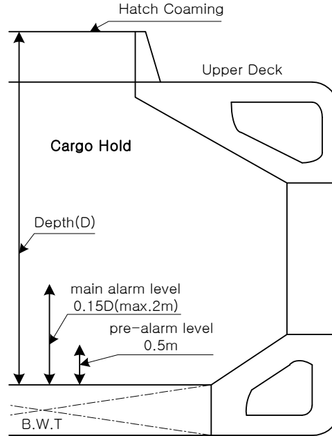
그림 1 선박깊이(D)
