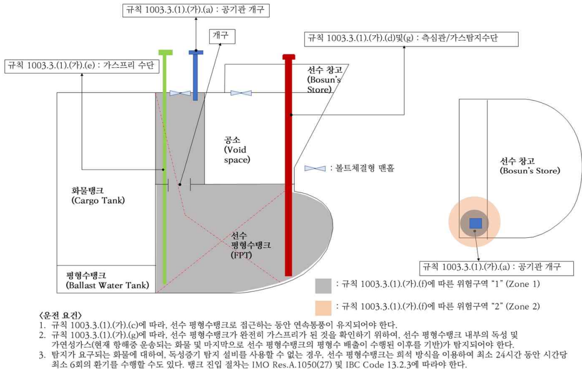
그림 7.1.32.4 유조선에만 적용가능한 배치의 예
