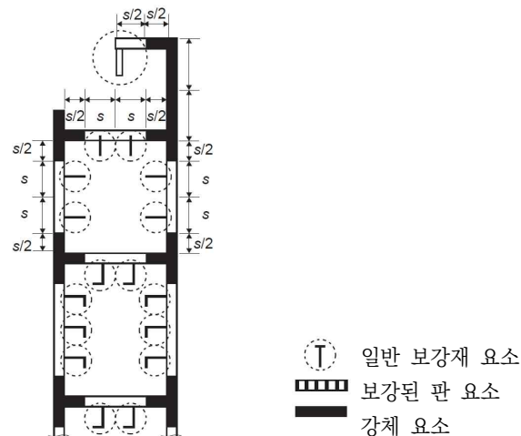
그림 A3.2 강체 요소 및 부착판 폭의 범위
