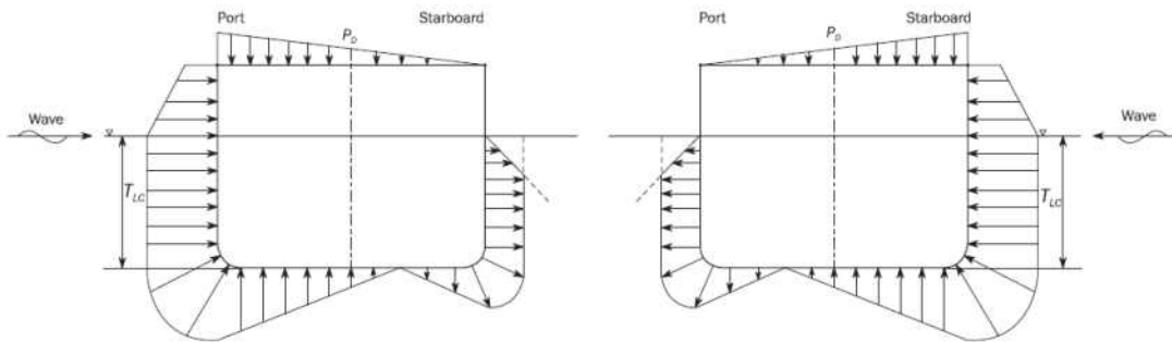
그림 14 BSR-2S (좌) 및 BSR-2P (우) 하중 상태에 대한 동적압력의 횡방향 분포
