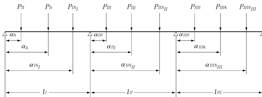
그림 7.7.5 P_{Ii}, \alpha_{Ii}, l_I 등의 측정방법
