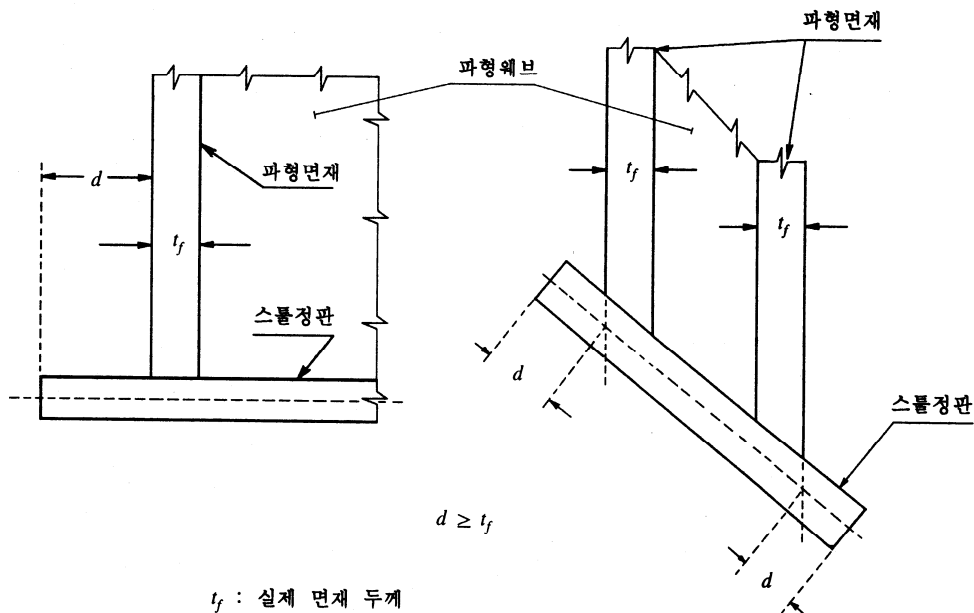
그림 7.3.18 스틸정판의 끝단으로부터 파형 면재까지의 허용 거리 d
