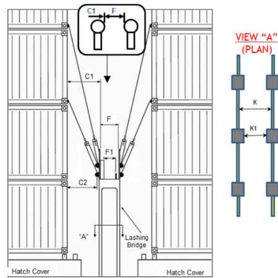
그림 2 Lashing bridge
