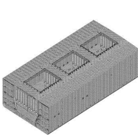
그림 3 중양부 화물창 모델그림
