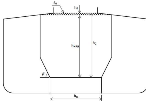
그림 4 화물창의 적재형상
