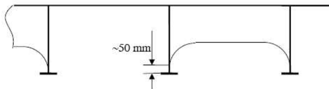
그림 7.3.9 트리핑 브래킷
