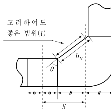
그림 7.10.3 S 의 측정방법
