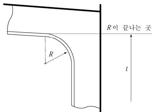
그림 7.10.5 l 의 측정방법
