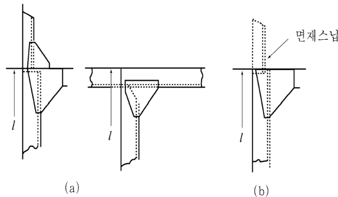
그림 5 끝부분의 고착
