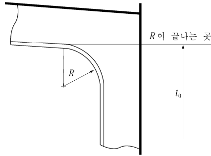
그림 7.1.19 l_0 의 측정방법
