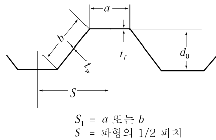
그림 6 S의 측정방법
