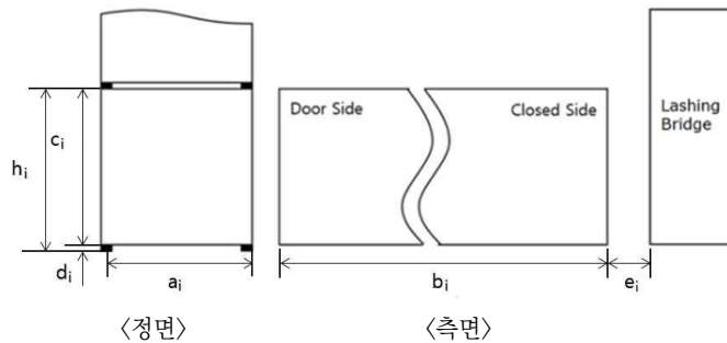
그림 5 컨테이너 주요치수
