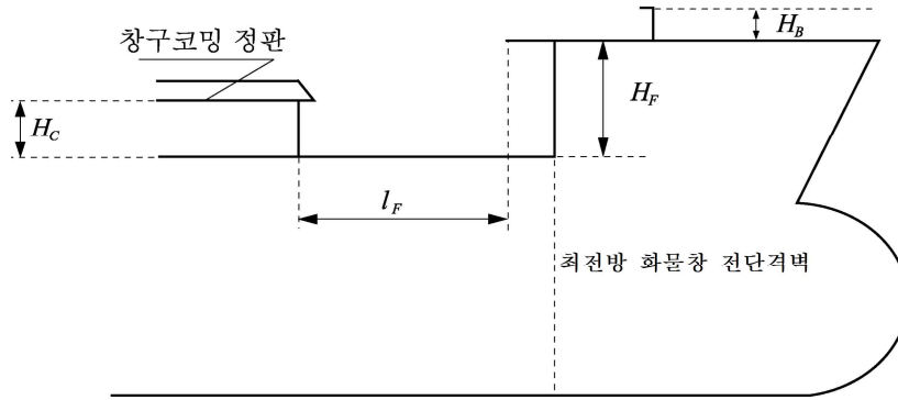
그림 7.3.21 선수루의 크기
