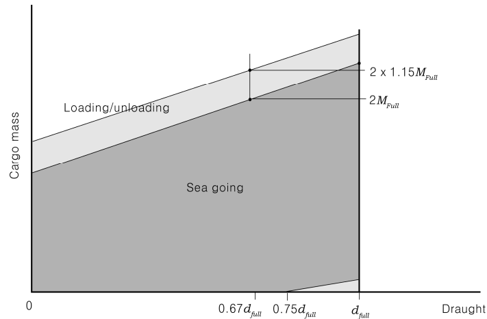
그림 2 두 개의 인접화물창의 최대허용 및 최소필요 화물질량(예)
