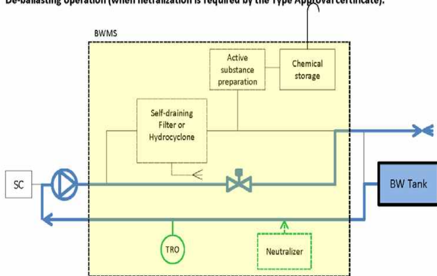
그림 8 평형수처리장치의 형식 6
