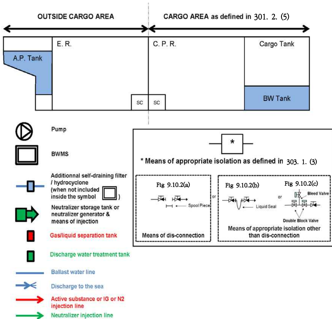
그림 9.10.4 배치도 예시
