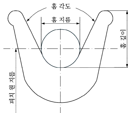
그림 9.2.8 시브그루브
