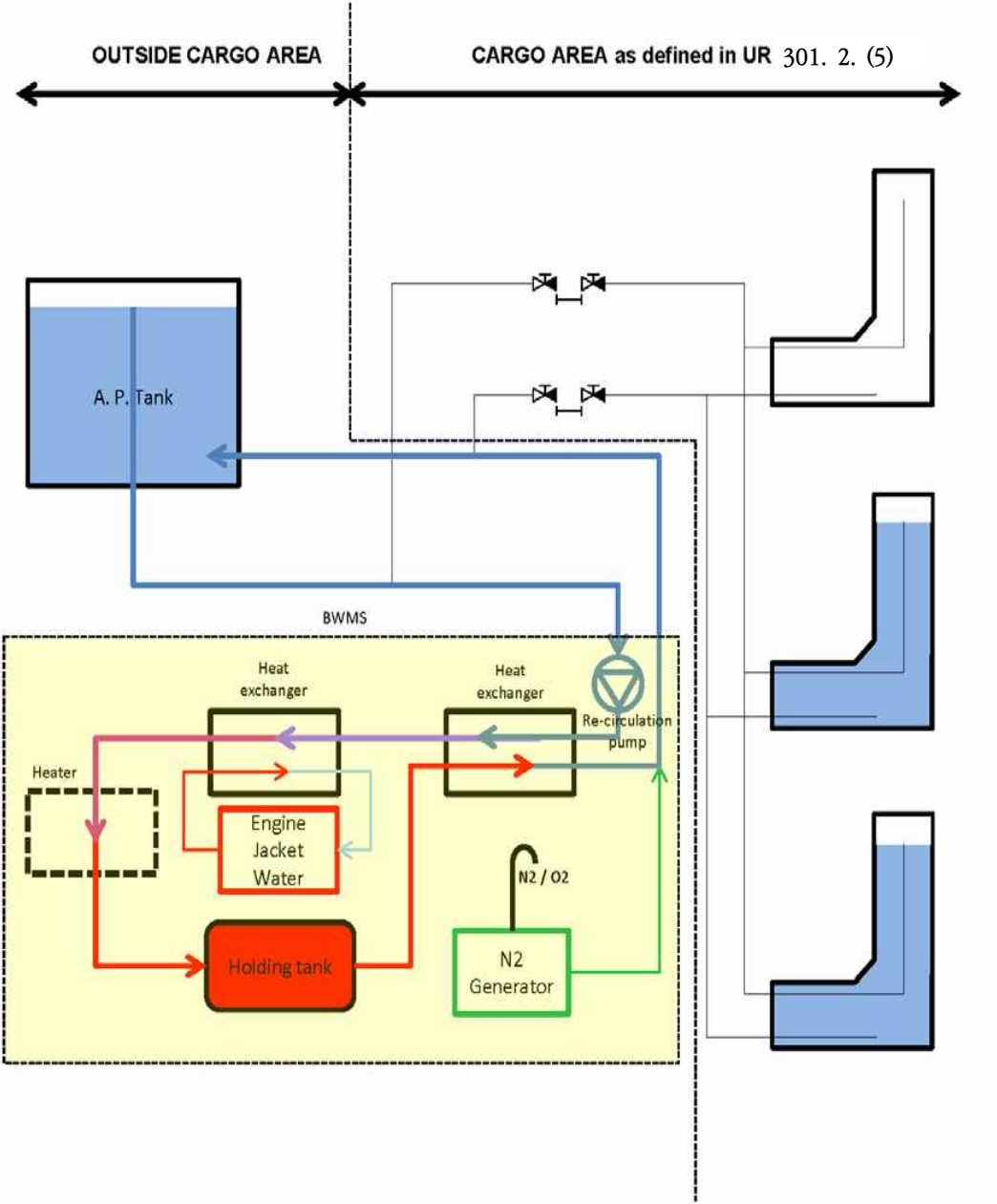
그림 11 평형수처리장치의 형식 8
