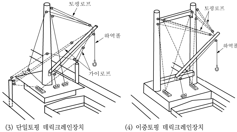
그림 9.2.1 데릭장치
