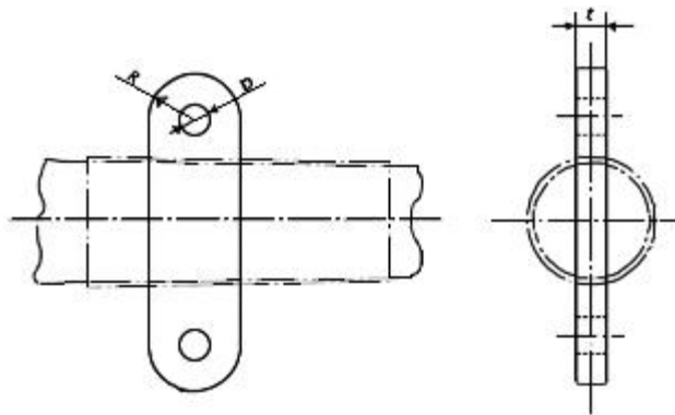
그림 9.2.7 데릭붐 정부에 부착되는 하역부속장구
