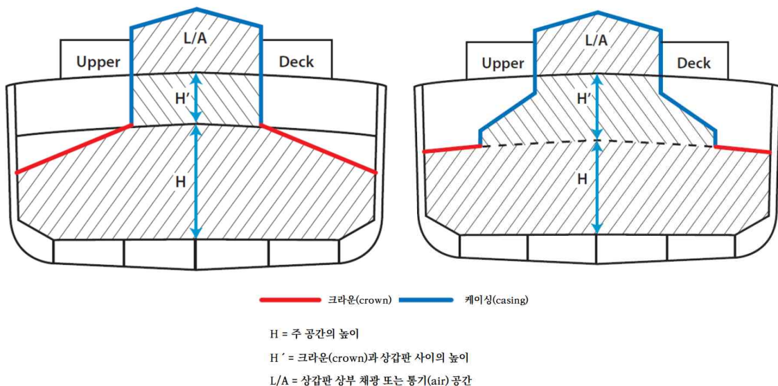
그림 8.9.1 A류 기관구역의 크라운(crown)
