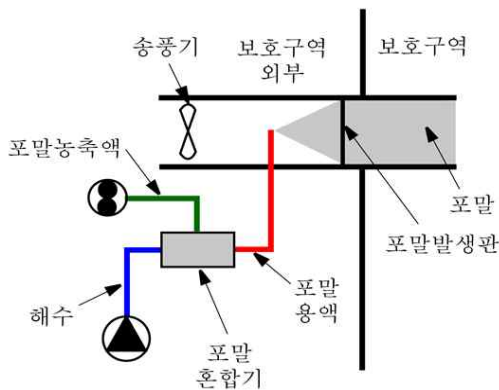
그림 8.8.5 외부공기식
