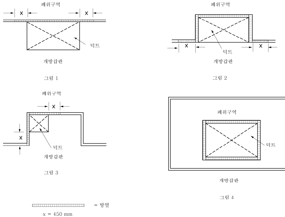
그림 8.7.6 패위구역에 인접하는 덕트의 예
