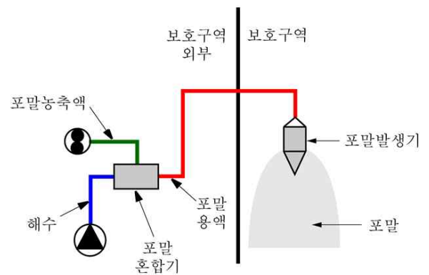
그림 8.8.6 내부공기식
