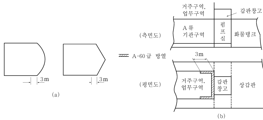
그림 8.7.3 화물지역에 인접하는 선루 및 감판실의 방열
