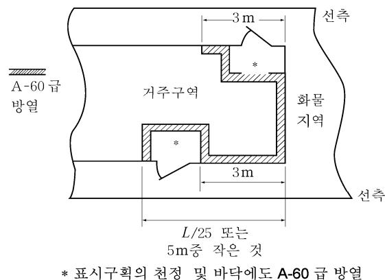
그림 8.2.7 A-60급 방열이 필요한 장소의 경계
