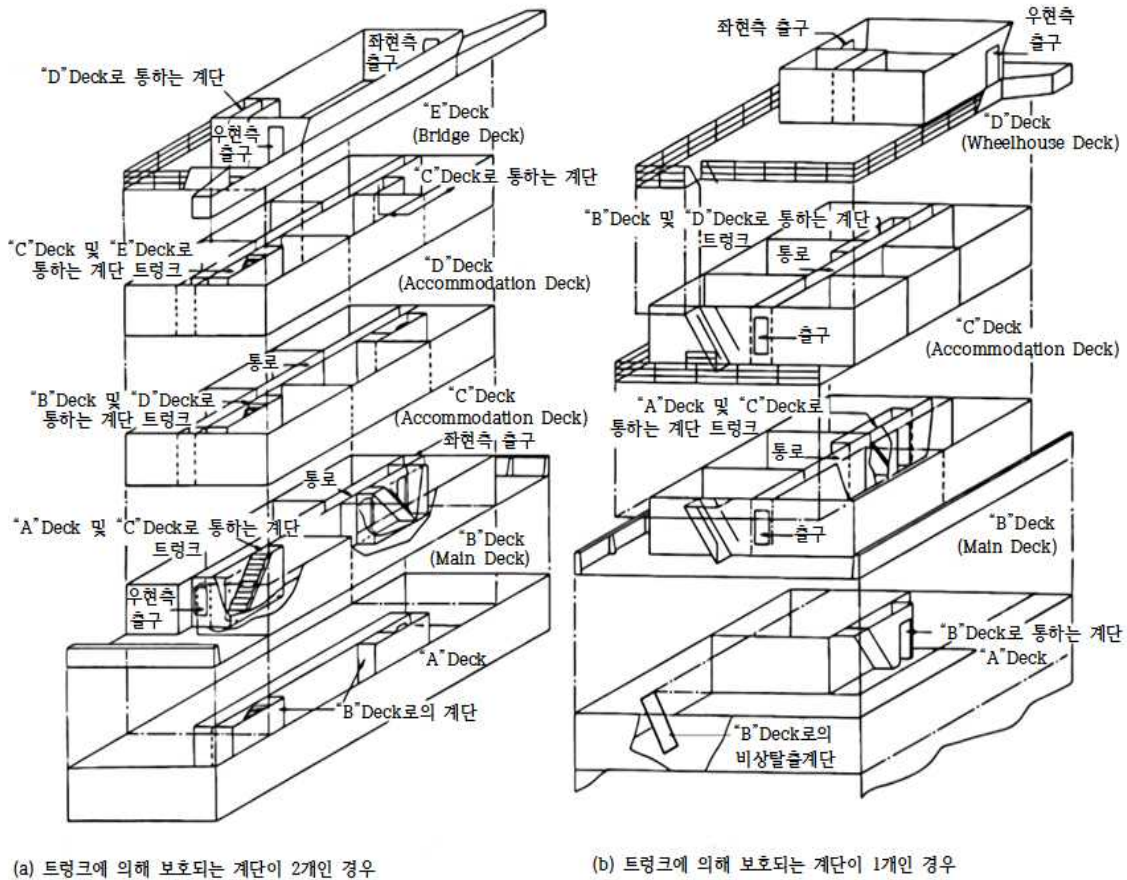
그림 8.10.1 탈출 설비
