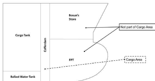
그림 8.1.1 화물지역의 배치 예제 (2026)
