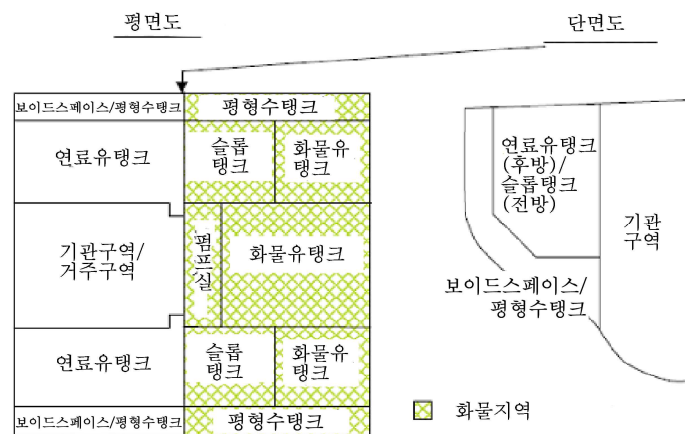
그림 8.2.2 화물유탱크의 격리
