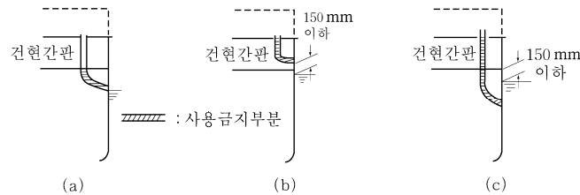
그림 8.9.2 열에 약한 재료의 사용이 금지되는 부분
