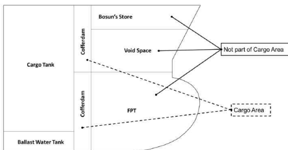
그림 8.1.1 화물지역의 배치 예제 (2026)
