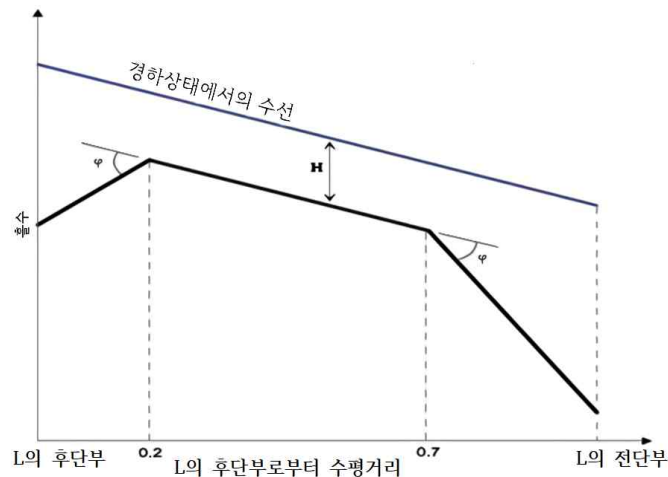
그림 8.8.1 종동요와 결합된 상하동요를 고려한 수선
