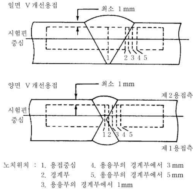
그림 7.5.18 용접 시험편의 노치위치
