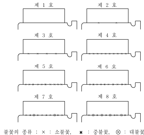
그림 6.1.5 정류자 표면의 불꽃 발생
