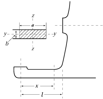
그림 10.2.1 슈퍼스의 좌표
