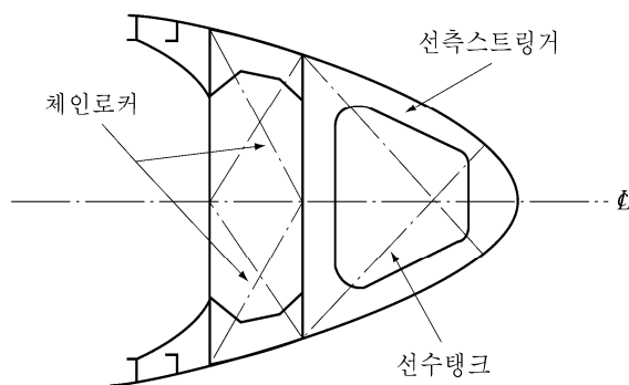
그림 10.13.1 체인로커부근의 선수구조
