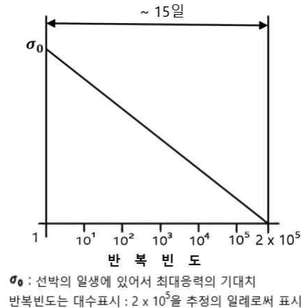
그림 6.3 간소화된 하중 분포
