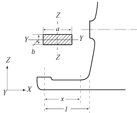
그림 3.2.1 슈피스의 좌표
