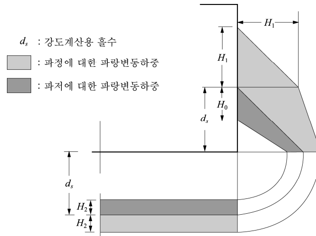
그림 5 파랑변동하중
