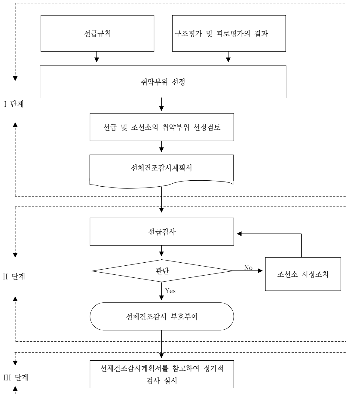
그림 1 선체건조감시절차
