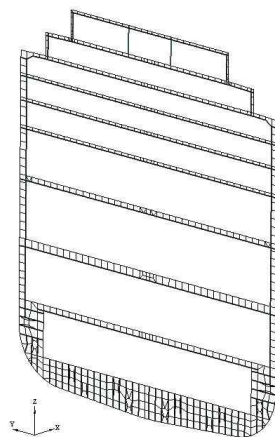
그림 28 특설늑골의 예
