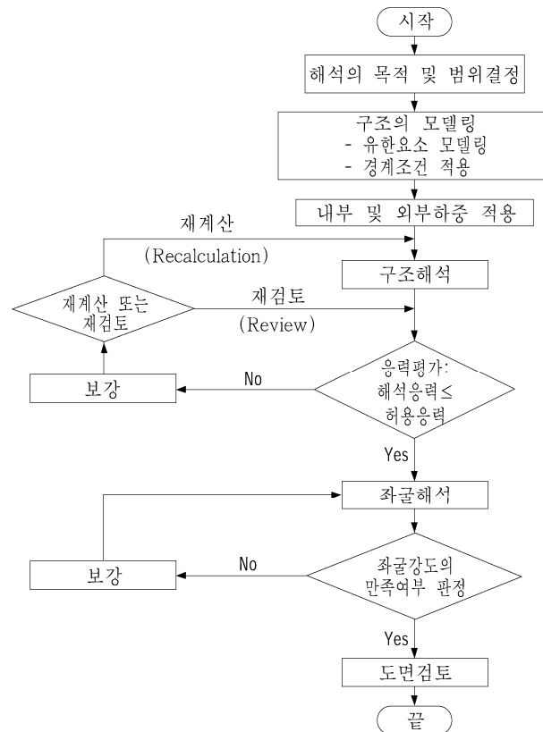
그림 4 화물창 구조해석 흐름도
