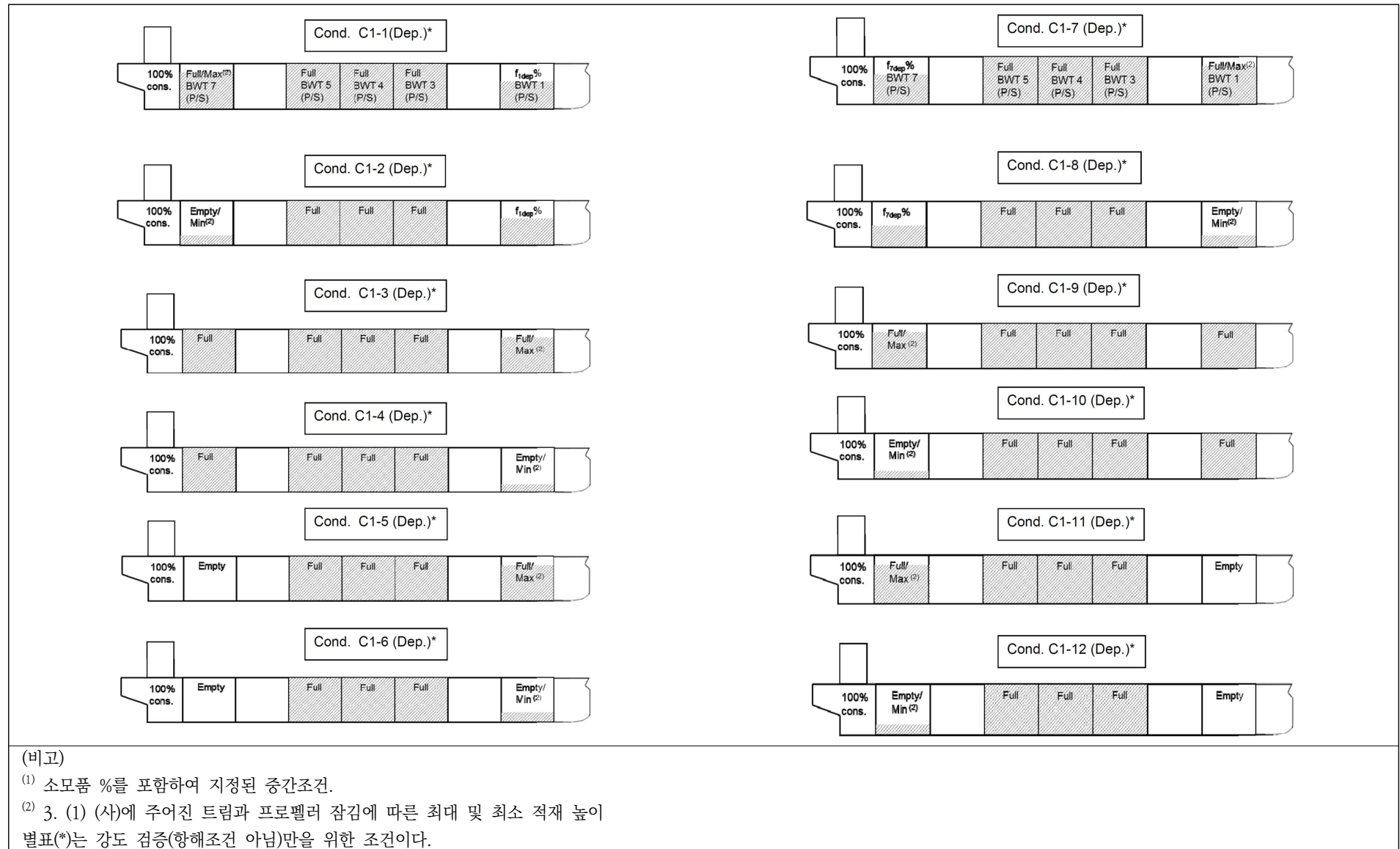
그림 7(b) 평형수 항해중 No.1 (P/S) 평형수 탱크와 No.7 (P/S) 평형수 탱크 모두 부분 적재를 하는 광석운반선의 하중조건 - Case C1
