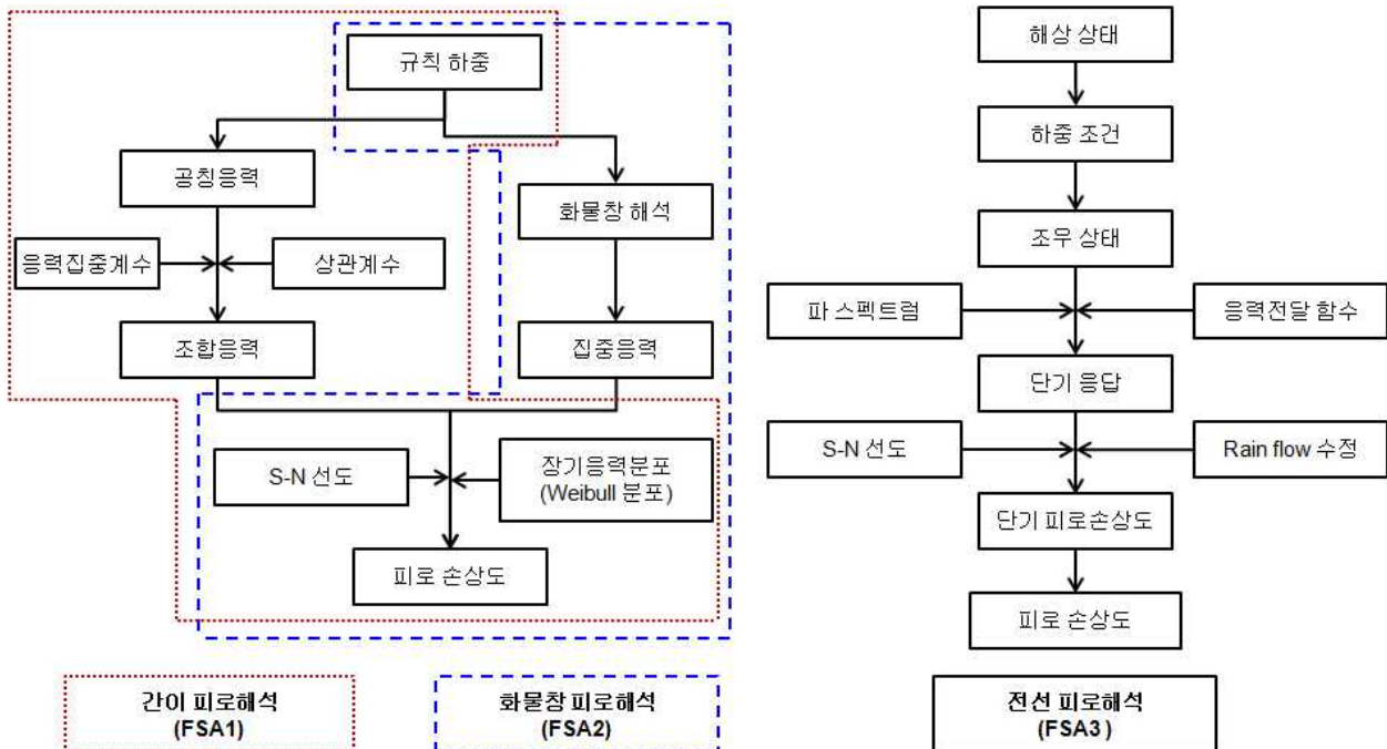
그림 1 피로해석 방법
