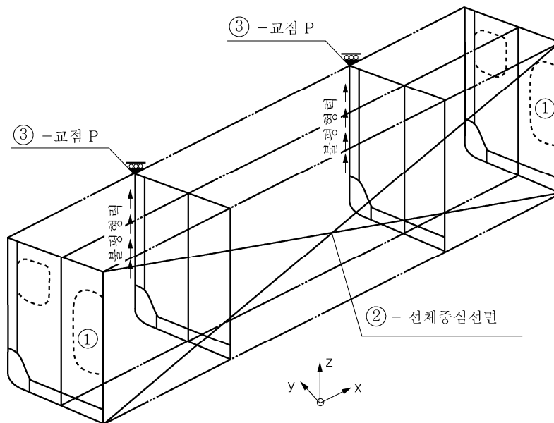
그림 18 경계조건 (대칭하중)
