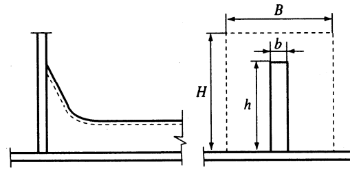
그림 3.5.15 유효접착면적
