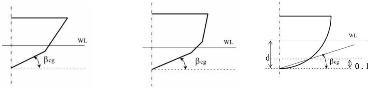
그림 3.2.4 선저각도, \beta_{cg}
