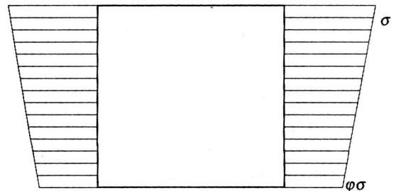
그림 3.2 좌굴응력 보정계수
