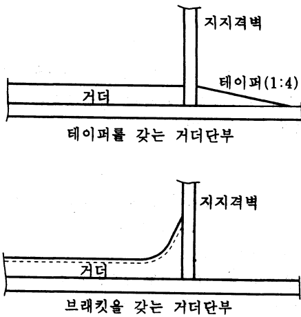
그림 3.5.11 거더의 단부
