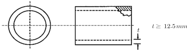
그림 1.5.6 원통형 관망창
