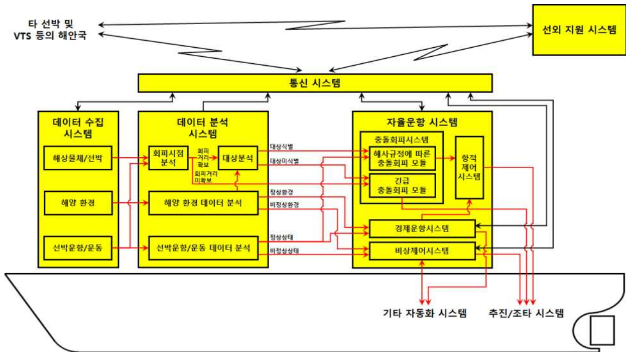
그림 3.1 자율화시스템의 일반적인 구성
