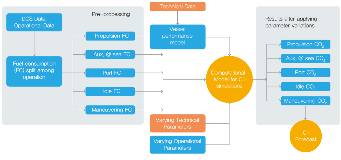
예시 3) 선박 성능 모델에서 운항 데이터, 흘수, 속도, 날씨(AIS 및 과거 해상 데이터)를 선박의 기술적인 인자와 결합하여 평가
