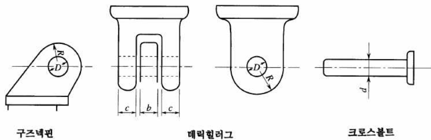
그림 9.2.5 구즈넥핀, 데릭힐러그 및 크로스볼트
