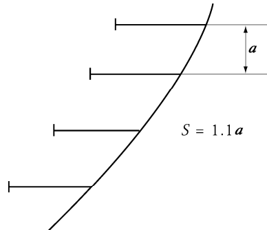
그림 10.4.1 선수미부에서의 S 와 a 와의 관계
