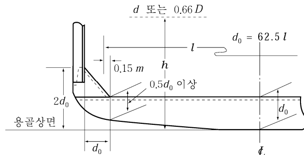
그림 10.6.1 늑판의 모양
