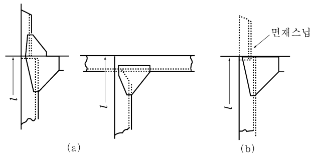
그림 10.14.1 끝부분의 고착 방법
