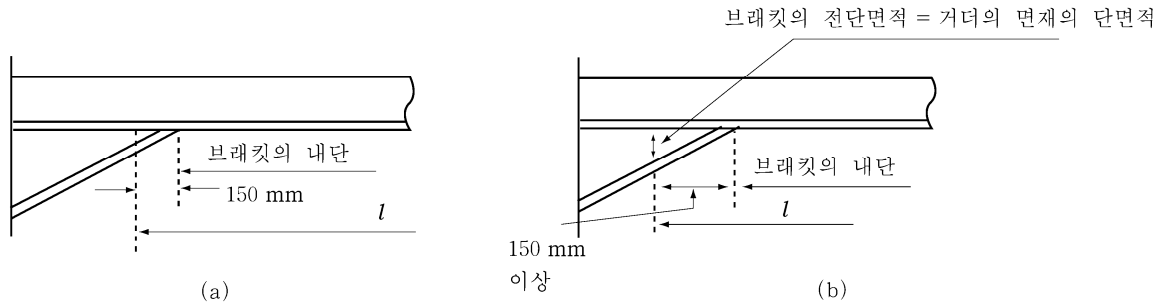
그림 10.1.2 l 의 수정
