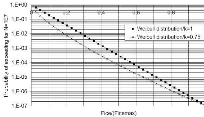
그림 1.10 피로설계에 사용되는 Weibull-type 분포(Fice가 (Fice)max를 넘을 가능성)
