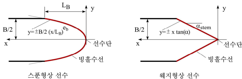
그림 2.7 선수형상 정의
