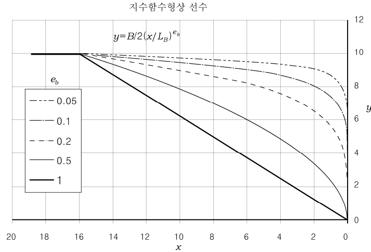
그림 2.8 B=20 이고 L_B=16 인 선수형상에 대한 e_b 영향의 도식
