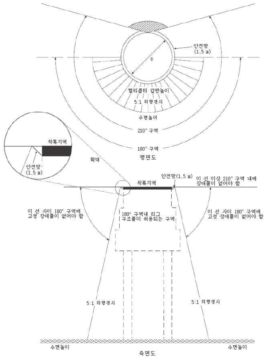
그림 12.1 무장애물 구역 - 착륙지역 하부
