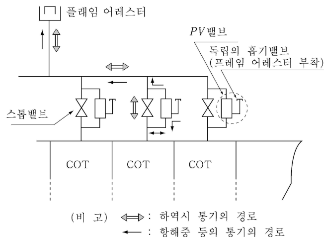
그림 8.2.8 화물유탱크 격리의 예
