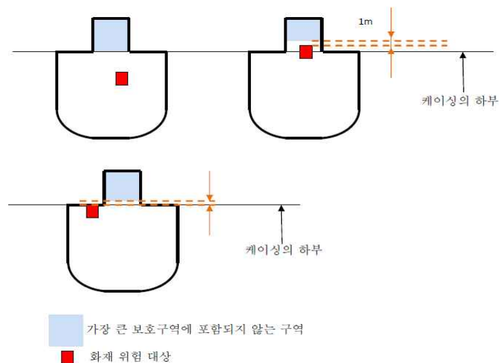
그림 8.8.3 엔진 케이싱이 있는 기관구역의 가장 큰 보호구역
