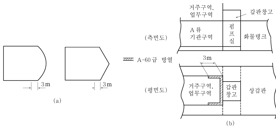
그림 8.7.2 화물지역에 인접하는 선루 및 갑판실의 방열
