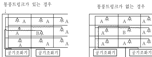
그림 8.7.5 폐위구역에 인접하는 덕트의 예
