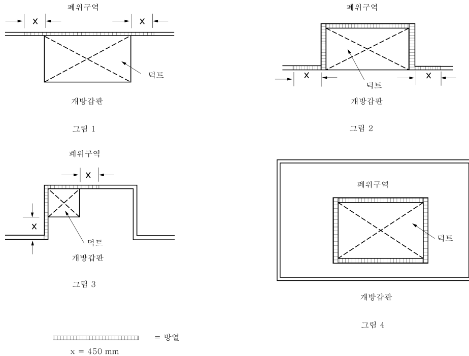
그림 8.7.5 폐위구역에 인접하는 덕트의 예
