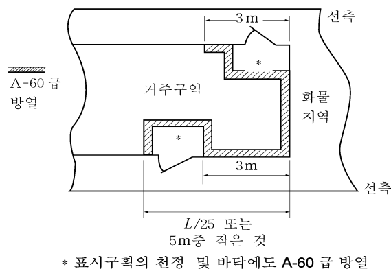
그림 8.2.7 A-60급 방열이 필요한 장소의 경계
