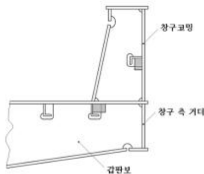
그림 4.2.12 코밍의 연장
