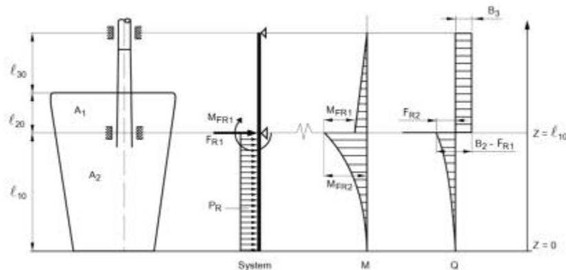
그림 4.1.3 트링크가 있는 스페이드 타 (2019)
