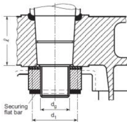
그림 4.1.7 키를 가지지 않는 콘커플링
