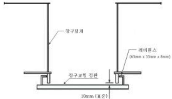
그림 4.2.14 레비린스의 예
