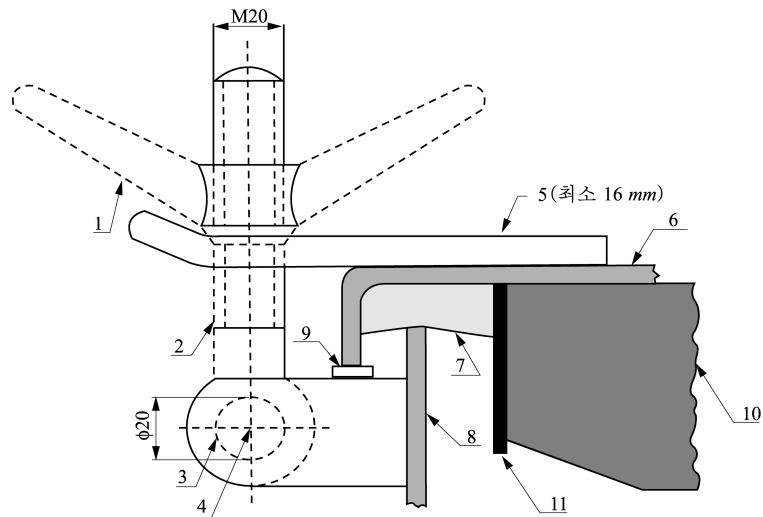
그림 4.9.1 보강재의 배치
