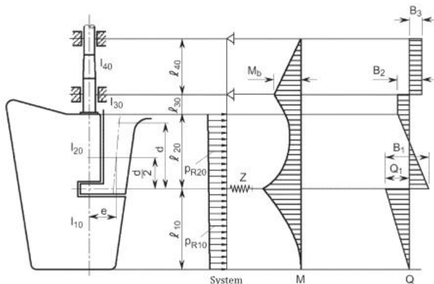
그림 4.1.5 D형 타(1점 탄성지지되는 세미스페이스드 타)
