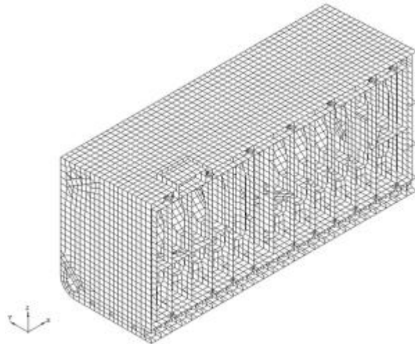
그림 51 화물창 모델 예(중앙부 화물창, 중심선 단면 표시)
