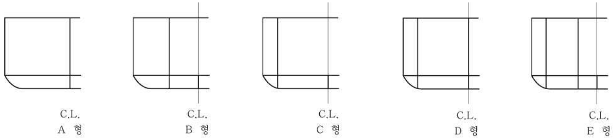
그림 3.3.7 종격벽 배치에 따른 선박의 분류
