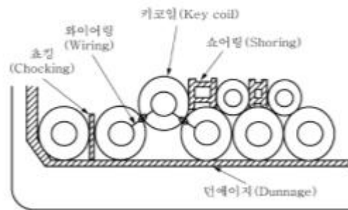
그림 1 강재코일 적재의 예
