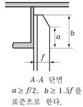
그림 3.7.8 스트럿과 종늑골의 겹침상세
