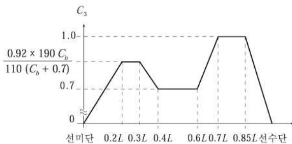
그림 3.3.5 계수 C_3 의 값
