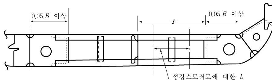
그림 3.7.1 조립늑판
