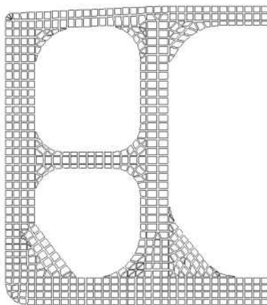
그림 17 Web frame 모델의 예
