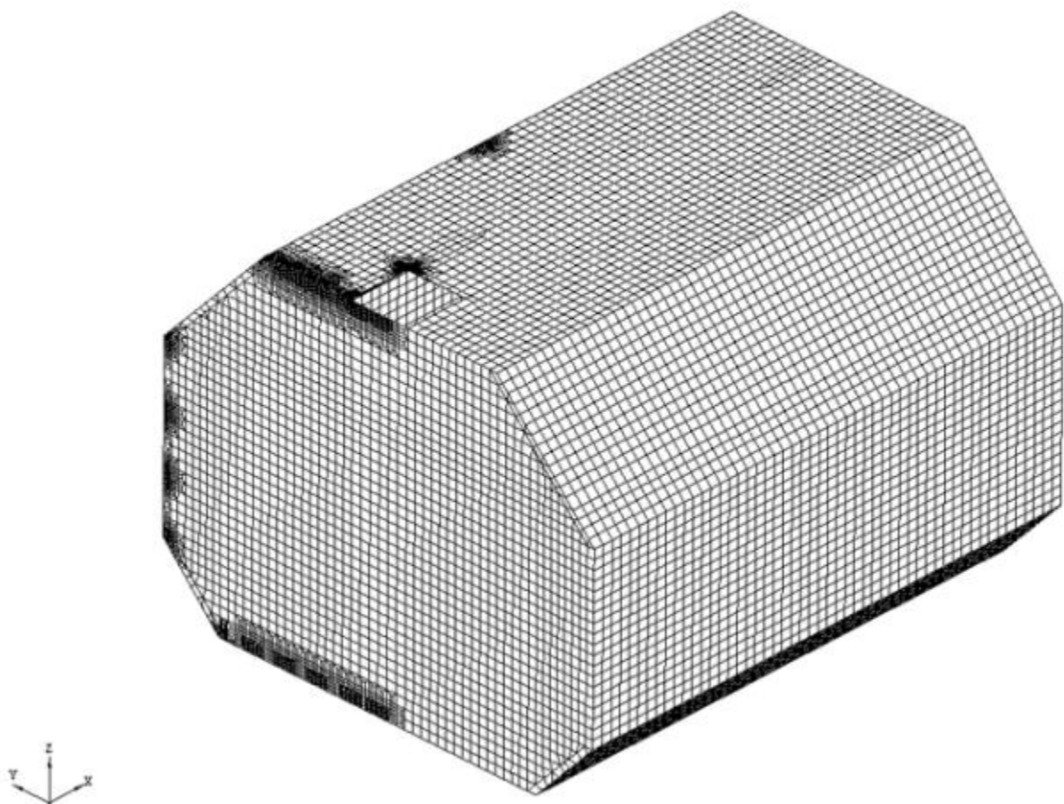
그림 40 상세 요소 분할의 예2
