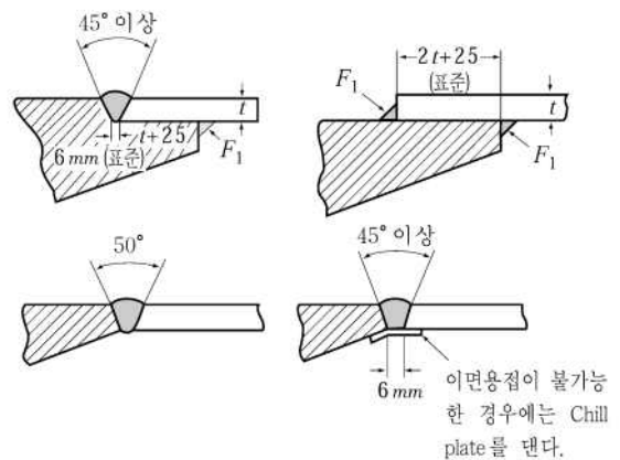
그림 3.2.2 주강선미재와 외판과의 고착
