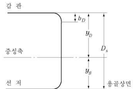
그림 3.1.6 갑판에만 고장력강을 사용하는 경우
