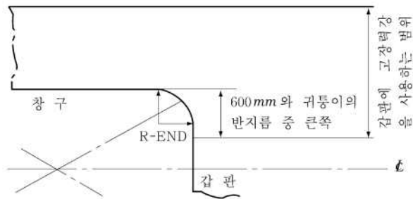
그림 3.1.7 갑판
