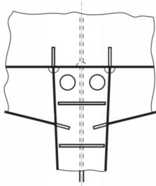
그림 3.2.6 러더혼과 선미구조의 결합
