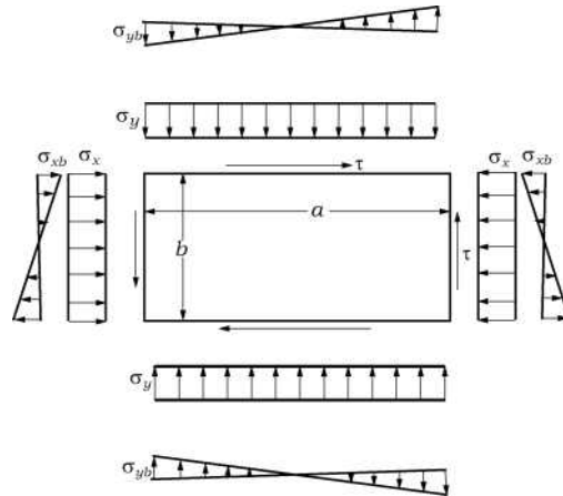
그림 6 패널의 작용응력
