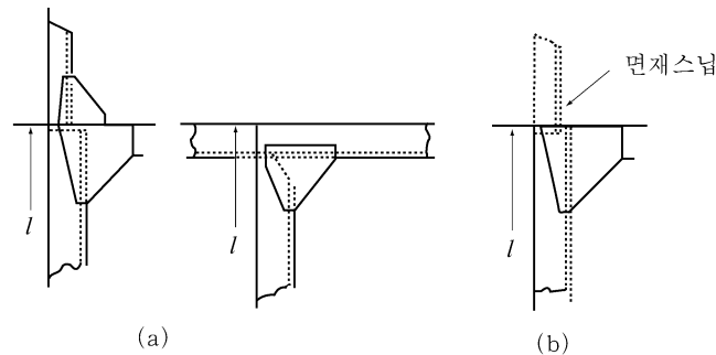
그림 3.14.2 끝부분의 고착
