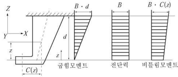
그림 3.2.2 러더혼의 하중
