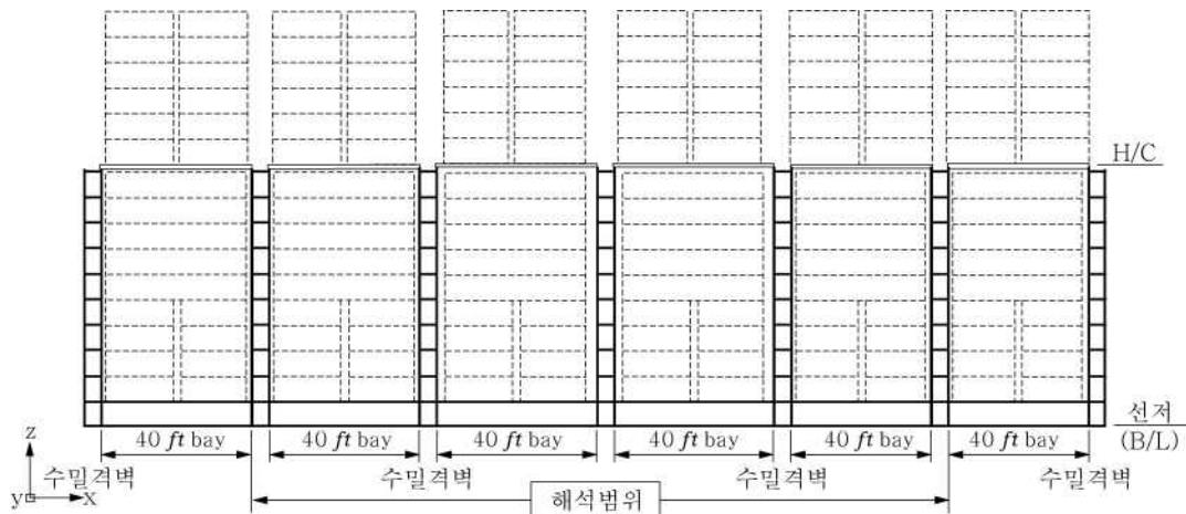
그림 19 해석범위
