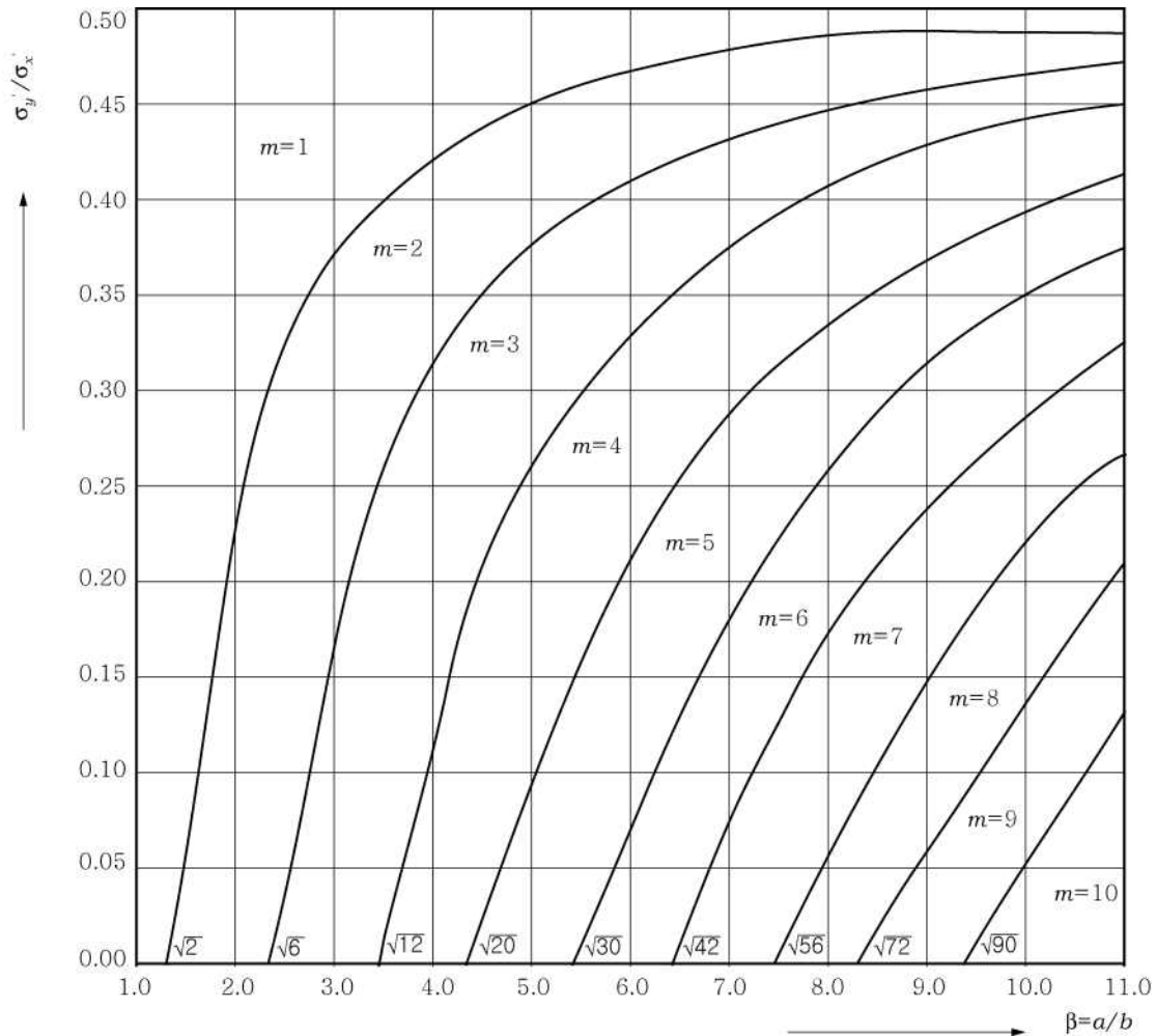
그림 7 최소 좌굴 응력하의 좌굴형상의 반파장수
