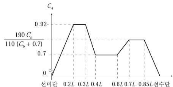
그림 3.3.6 계수 C_4 의 값
