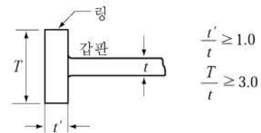
그림 3.3.4 링에 의한 보강
