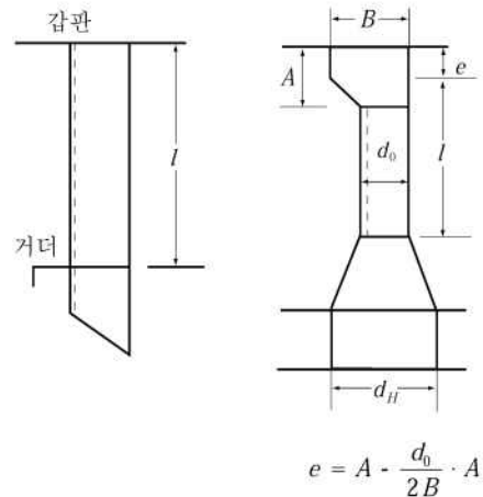
그림 3.15.1 l의 측정방법
