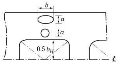
그림 3.3.3 타원형과 원형 개구가 동일단면상에 있는 경우
