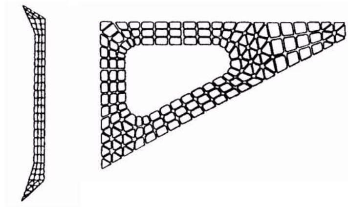
그림 12 상세분할 해석에 의한 모델의 예
