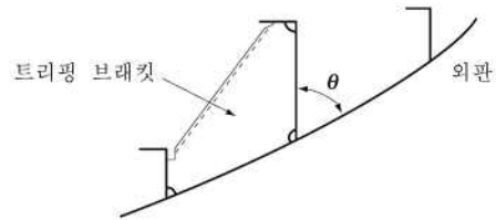
그림 3.13.1 거더 웹과 외판이 이루는 각이 작은 경우
