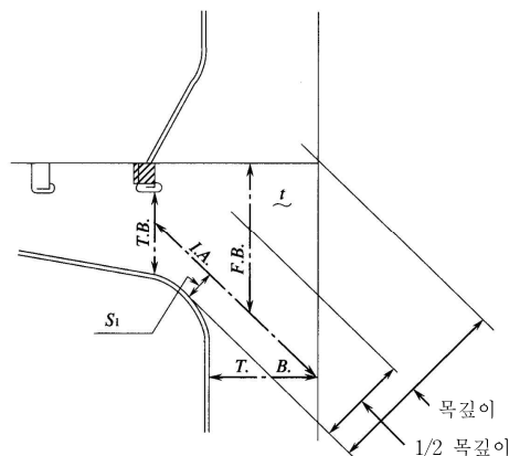
그림 3.9.4 브래킷의 보강
