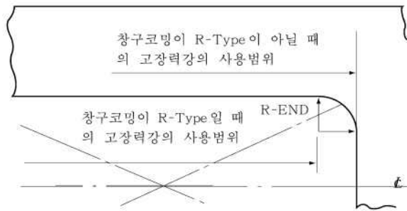
그림 3.1.8 창구코밍
