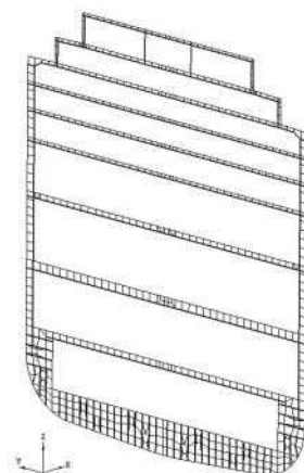
그림 28 특설늑골의 예
