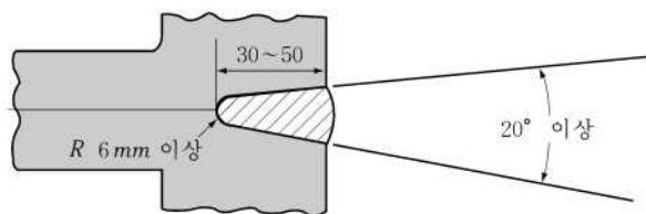
그림 3.2.1 주강선미재의 상호 용접이음
