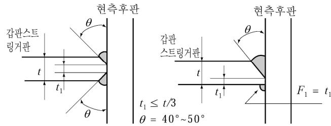
그림 3.4.1 현측후판과 갑판스트링거판 결합부의 용접상세
