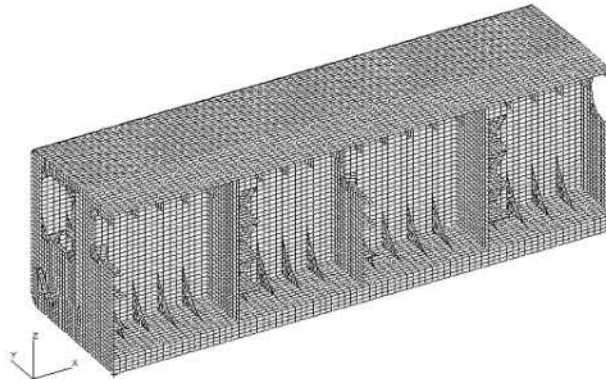
그림 16 화물창 모델의 예
