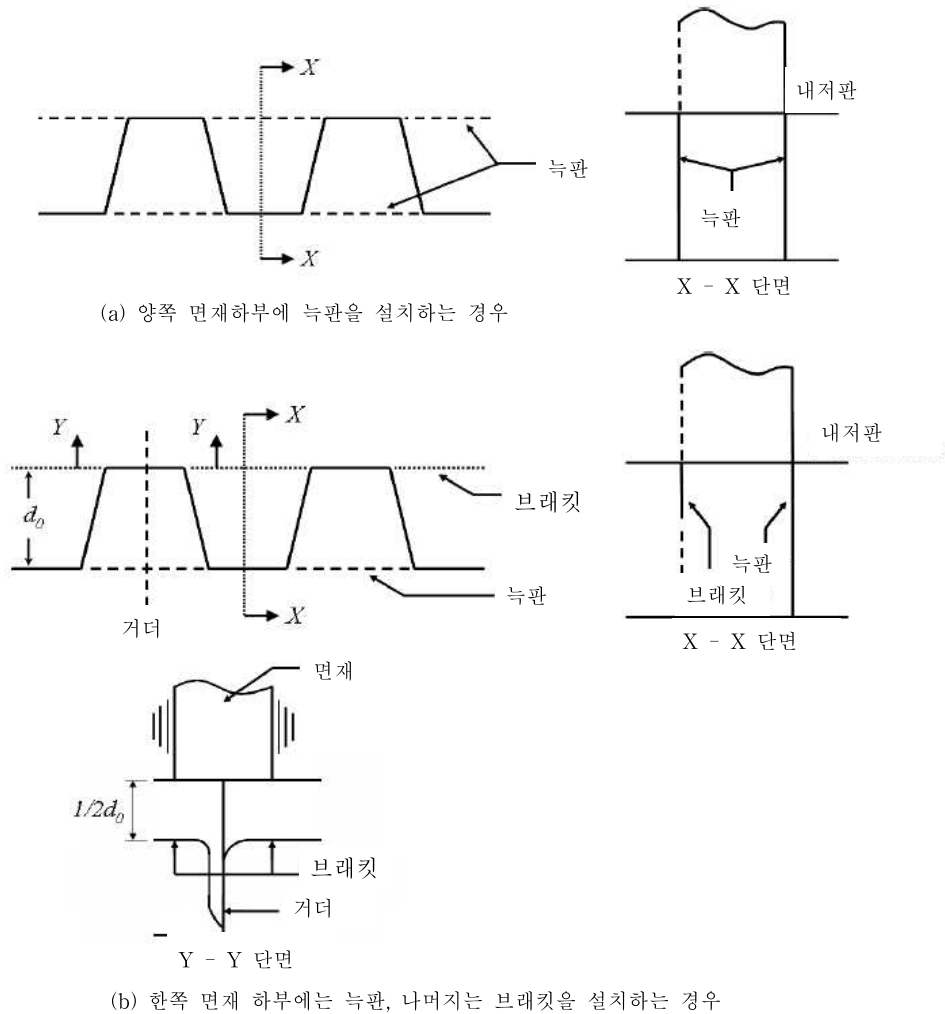
그림 3.15.2 파형격벽을 지지하는 구조의 예(횡격벽)
