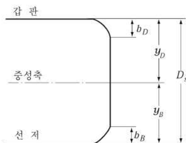
그림 3.1.5 갑판과 선저에 고장력강을 사용하는 경우
