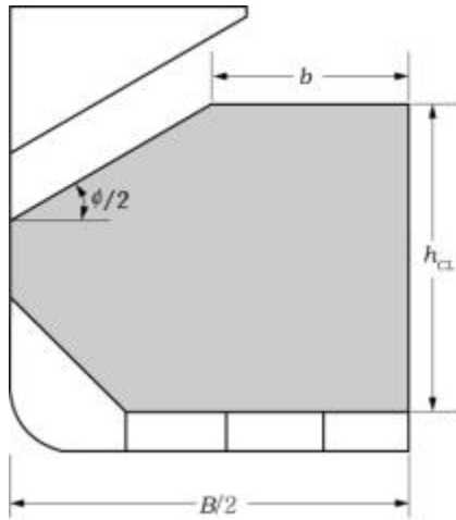
그림 14 화물창의 적재형상
