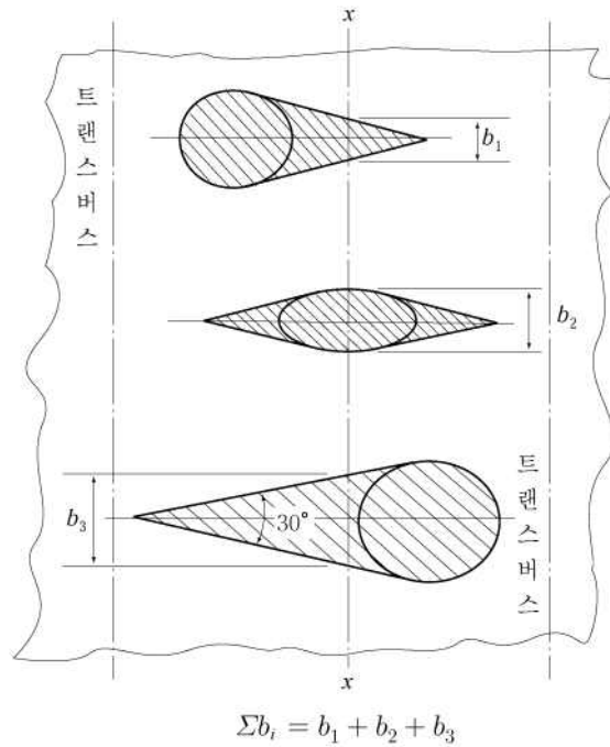
그림 3.3.3 강력갑판상의 개구
