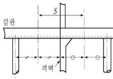
그림 3.14.2 S의 측정방법
