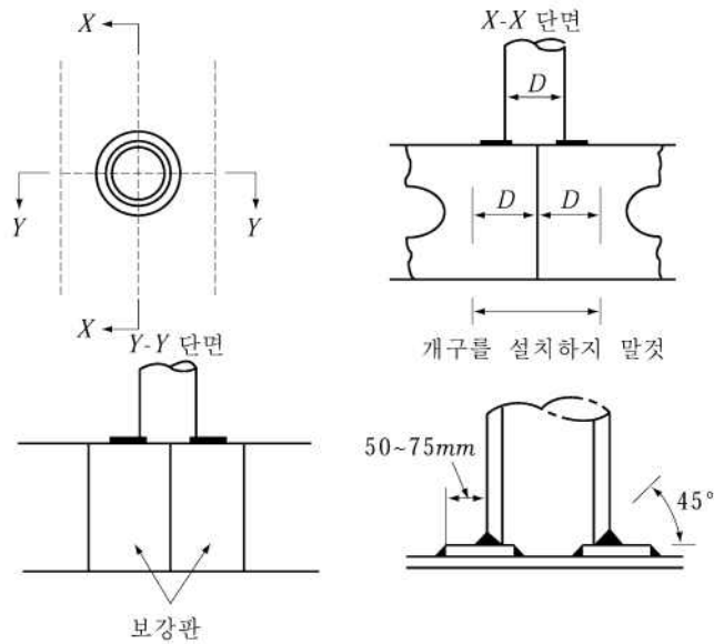
그림 3.12.1 필러 하부의 보강
