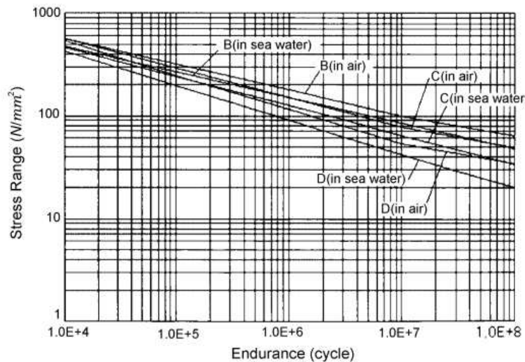
그림 2 설계 S-N 선도 *1
