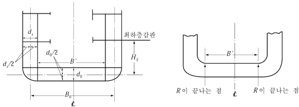
그림 3.7.5 이중 선측구조
