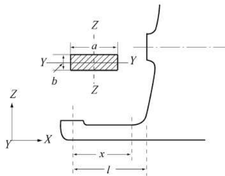
그림 3.2.1 슈피스의 좌표
