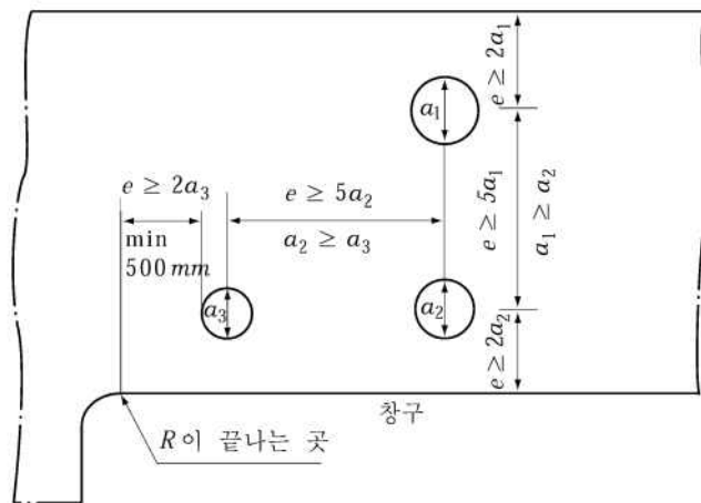
그림 3.3.5 개구의 간격
