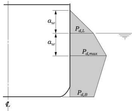
그림 3 국부 파랑압력범위 p_d
