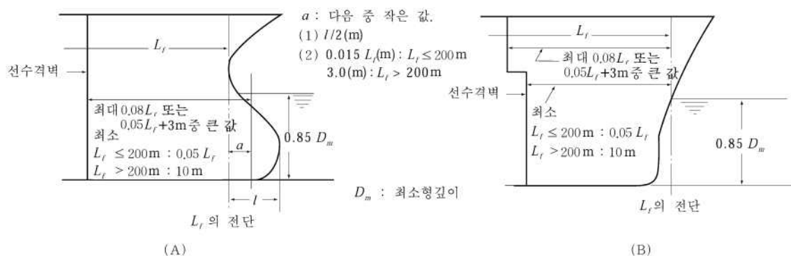
그림 3.14.1 선수격벽의 위치측정방법
