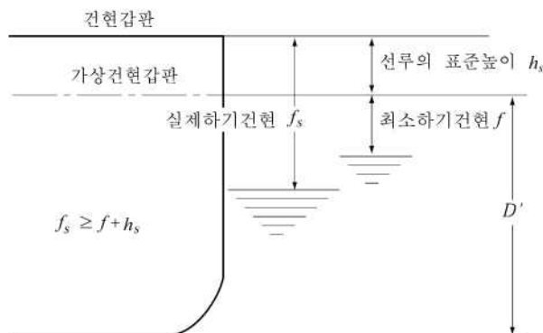
그림 3.1.4 특히 큰 건현을 가진 선박
