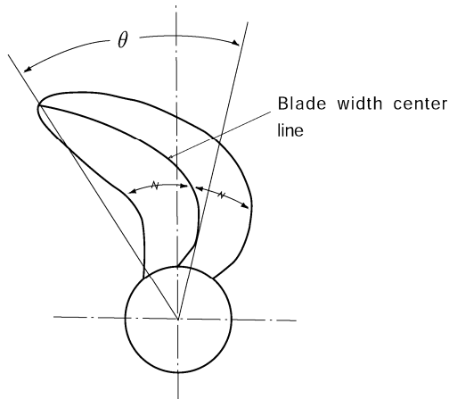
Fig 5.3.2 Skew Angle
