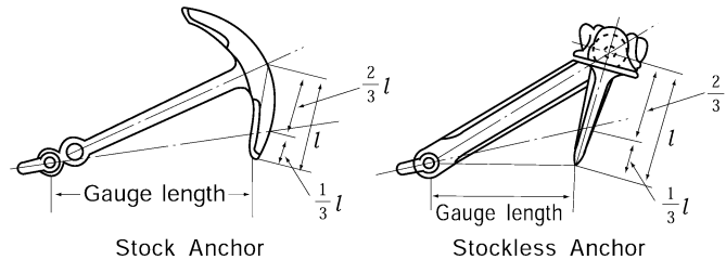
Fig 4.8.1 Anchors
