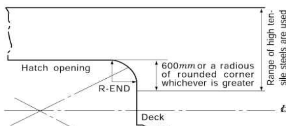
Fig 3.1.7. Deck
