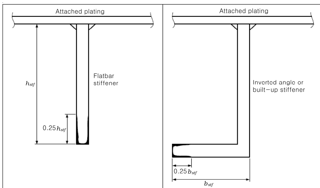
Fig 1.2.2 Edge corrosion
