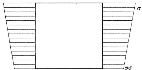
그림 3.2 좌굴응력 보정계수
