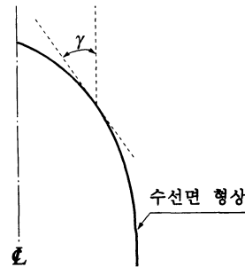
그림 3.2.7 각도 γ
