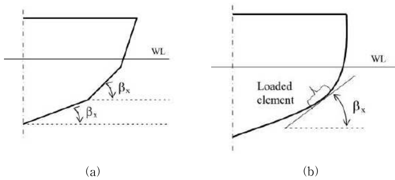
그림 3.2.4-1 \beta_X
