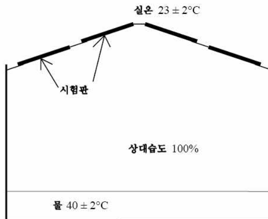
그림 3.30.3 응축체임버
