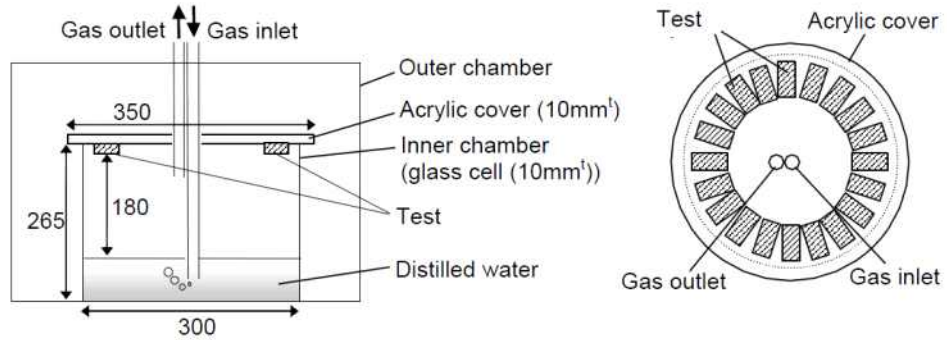
그림 3.32.2 상부압판 모의시험 장치의 예
