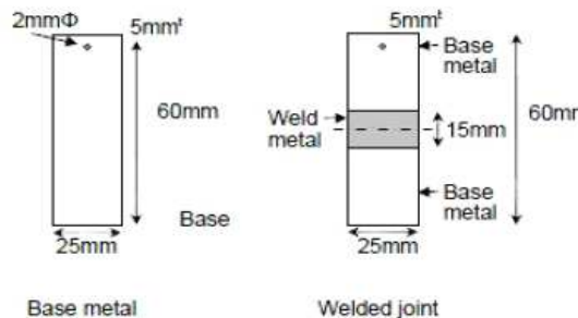
그림 3.32.5 시험재의 크기
