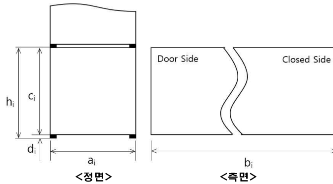
그림 3 컨테이너 주요치수
