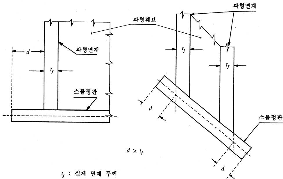
그림 7.3.18 스텔정판의 끝단으로부터 파형 면재까지의 허용 거리 d
