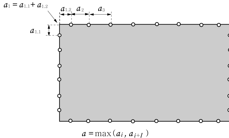
그림 7.3.8 고박장치의 간격
