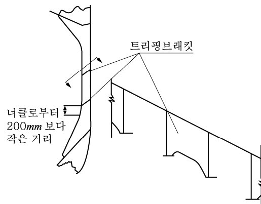
그림 7.3.25 트리핑 브래킷
