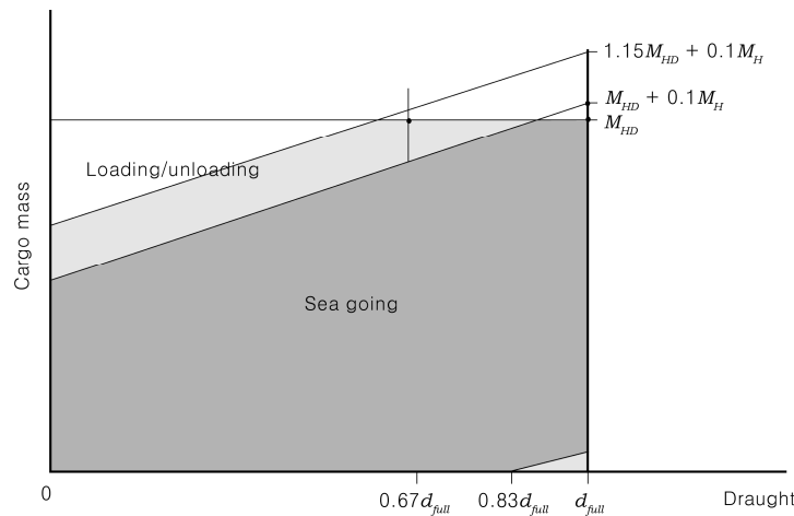
그림 1 단독화물창의 최대허용 및 최소필요 화물질량(BC-A 선박의 적하량의 예)
