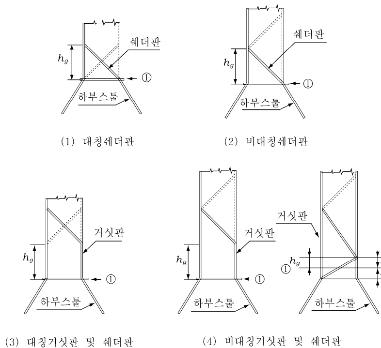
그림 4 데크판 및 거싯판
