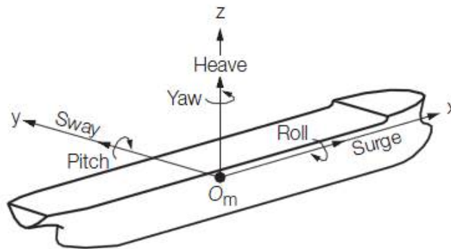
그림 2 운동 좌표계
