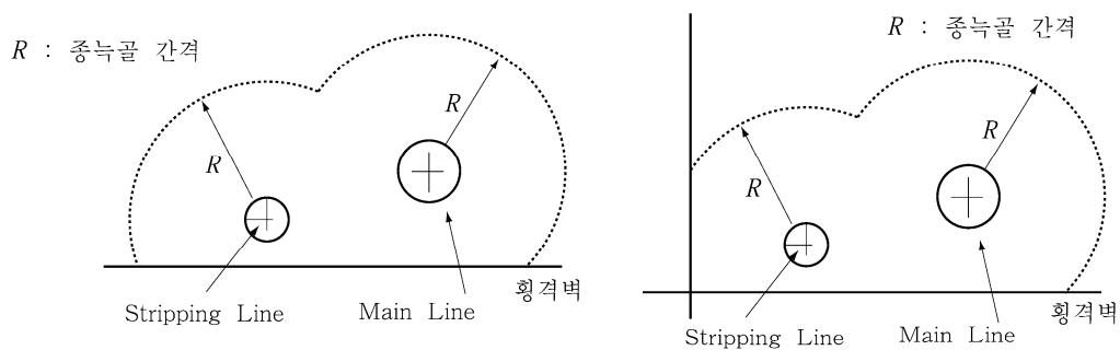
그림 7.10.14 내저판의 부식에 대한 보강 범위
