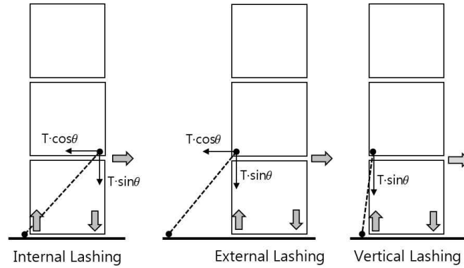
그림 7 래싱 방법의 종류
