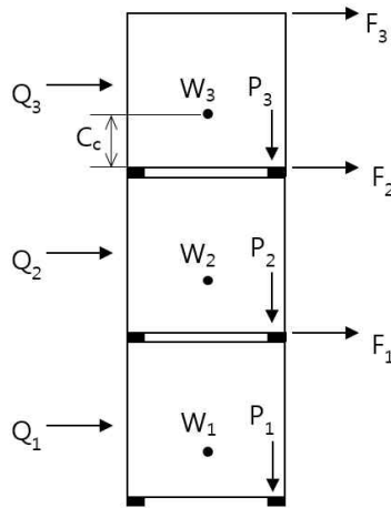
그림 4 래싱 하지 않은 스택에서 횡방향 하중의 계산 예
