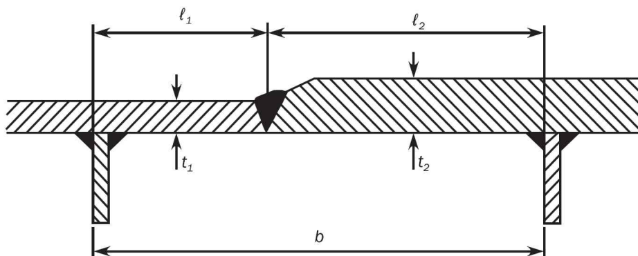
그림 A2.1 폭에 걸친 판 두께 변화
