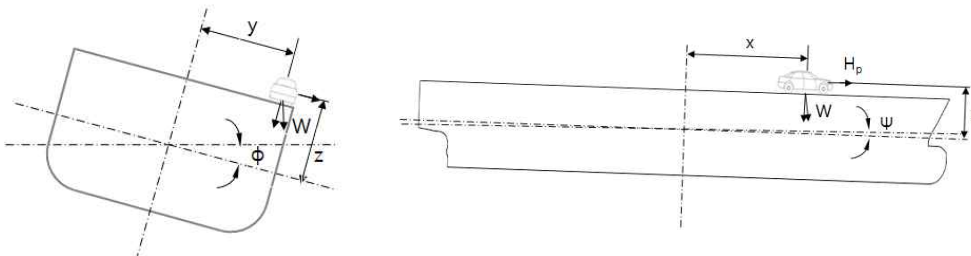
그림 1 선체운동
