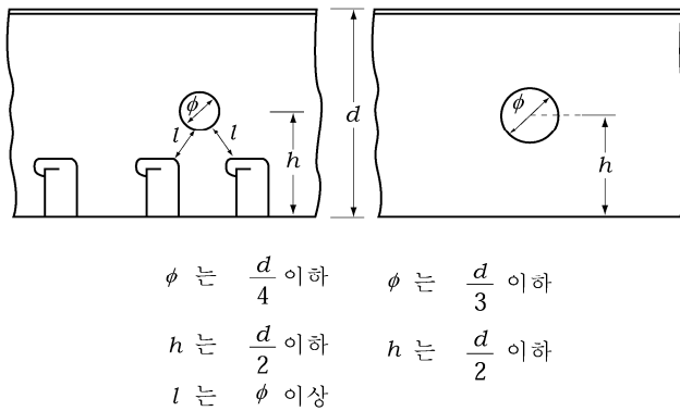
그림 7.1.16 경감구멍의 위치와 크기
