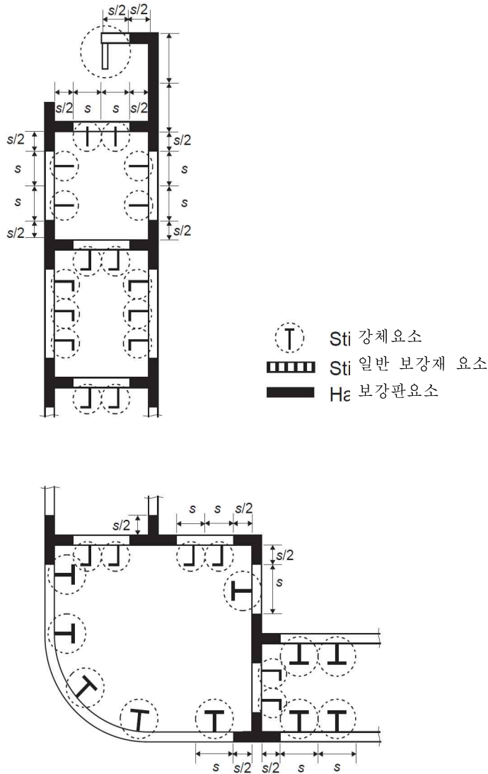
그림 A3.3 선체단면 보강판 요소, 일반 보강재 요소 및 강체 요소의 형상 예
