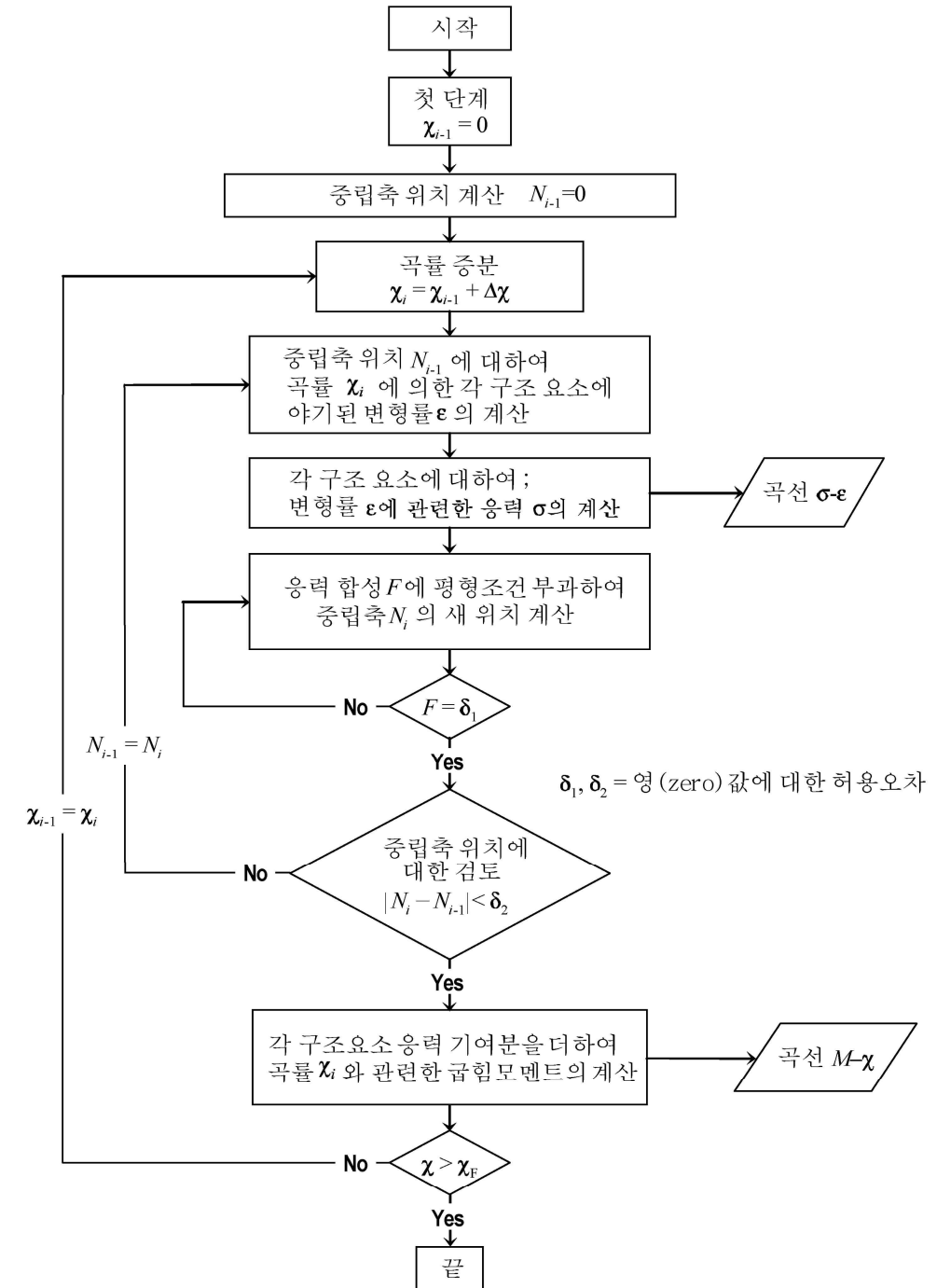
그림 A3.1 곡선 M-\chi 계산 과정 흐름도
