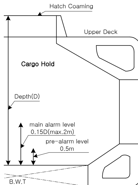
그림 1 선박깊이(D)
