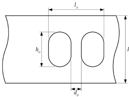
그림 7 웨브 내의 개구
