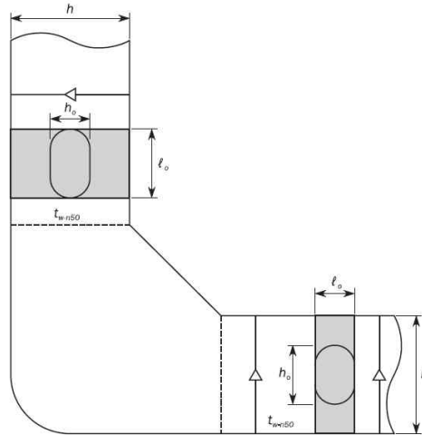
그림 6 웨브 내의 개구
