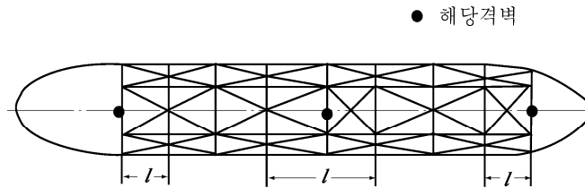
그림 7.1.5 l 의 측정방법
