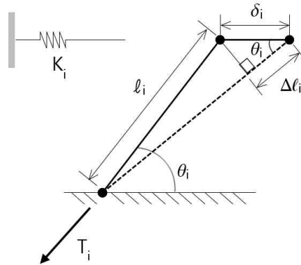
그림 5 래싱 설비의 수평 강성
