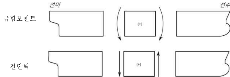
그림 7.4.4 굽힘모멘트 및 전단력에 대한 부호 규약
