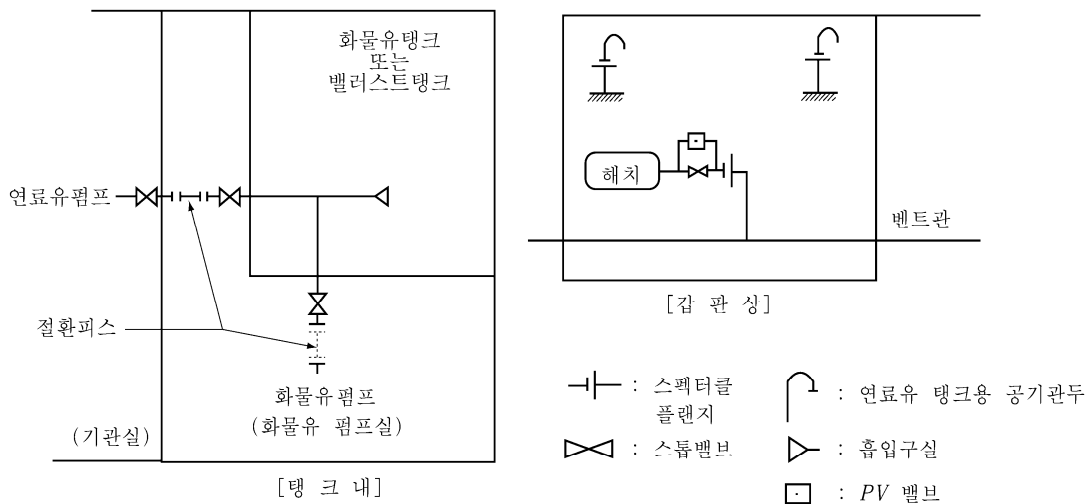
그림 7.1.32 화물유점 연료유택크의 배관 예
