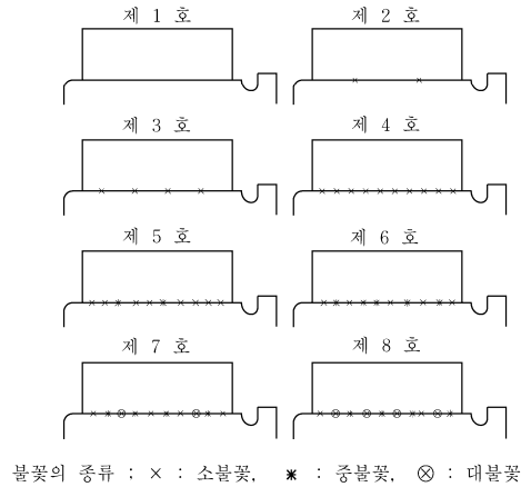
그림 6.1.3 정류자 표면의 불꽃 발생
