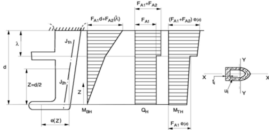
그림 4.1.8 러더혼
