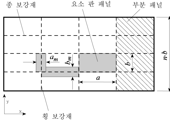
그림 4.2.7 패널의 일반적인 배치
