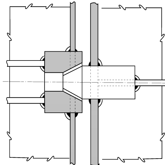
그림 4.3.4 추력베어링의 일례
