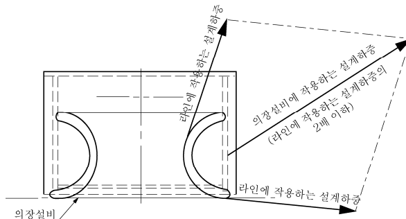
그림 4.10.1 설계하중의 적용
