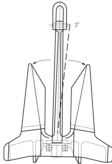
그림 4.8.2 앵커샹크의 경사 허용범위
