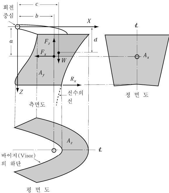
그림 4.3.2 상부 현지식 선수문 (bow visor)
