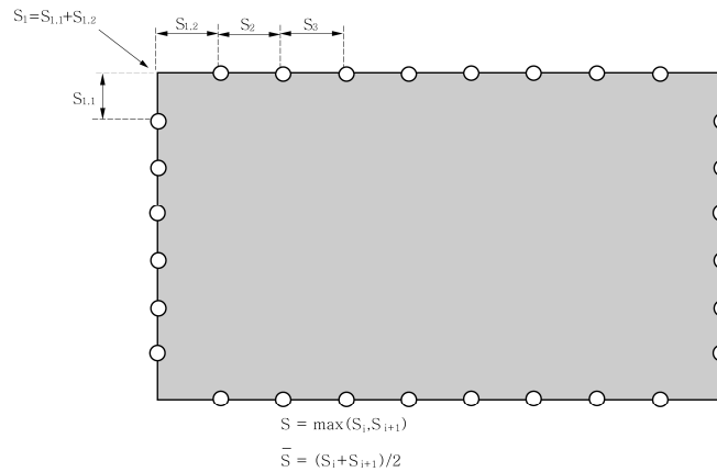
그림 4.2.5 고박장치의 간격
