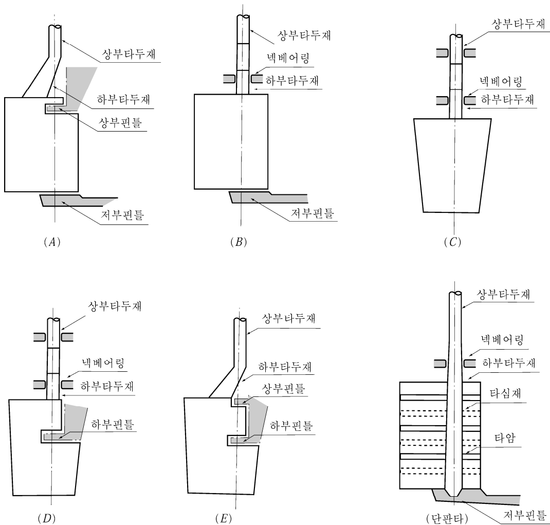
그림 4.1.1 타의 종류
