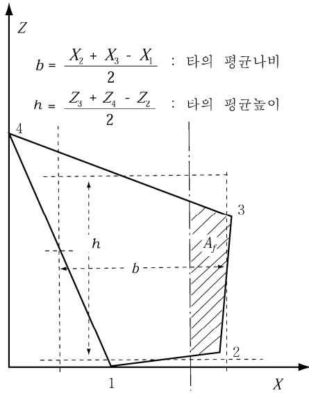
그림 4.1.2 타의 좌표계
