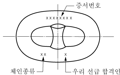
그림 4.8.6 체인의 표시
