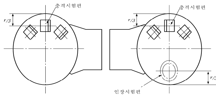
그림 4.8.11 체인 링크의 예
