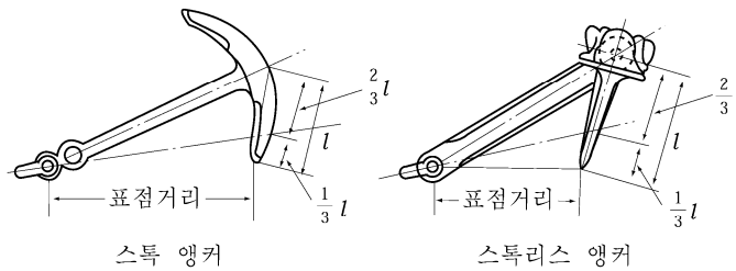
그림 4.8.1 앵 커
