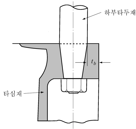
그림 4.1.2 하부타두재와 타십재의 커플링
