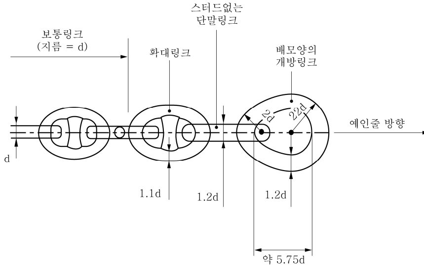
그림 4.8.10 마모방지 체인의 선외측 단부의 전형적인 배치
