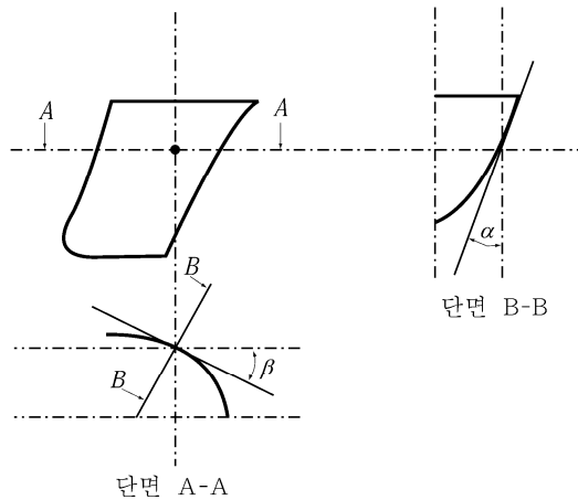
그림 4.3.1 플레어각 및 입수각
