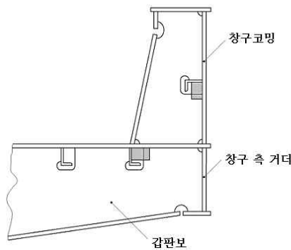
그림 4.2.12 코밍의 연장
