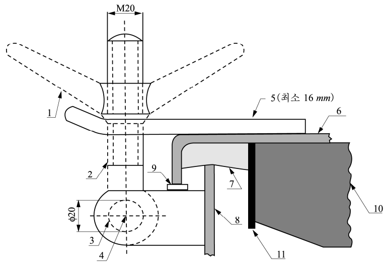
그림 4.9.1 보강재의 배치
