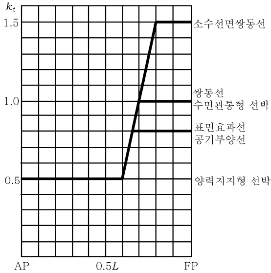
그림 3.2.7 쌍동선연결부 슬래밍 분포계수 k_t
