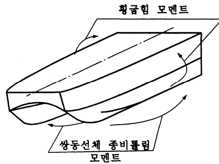
그림 3.2.13 쌍동선체 연결부의 종비틀림
