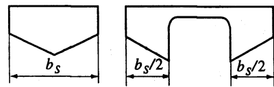
그림 3.2.11 중앙부 슬래밍 작용면적의 폭
