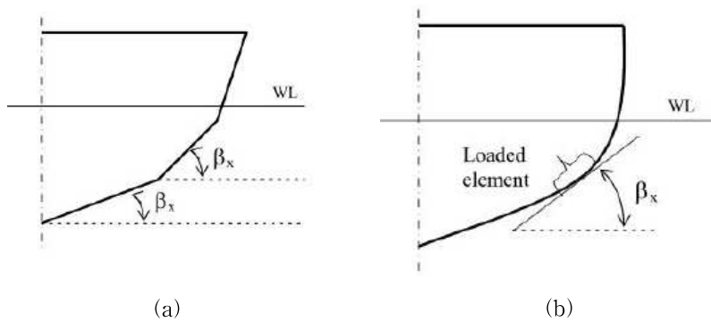
그림 3.2.4-1 \beta_X
