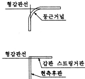
그림 3.3.3 형기준선
