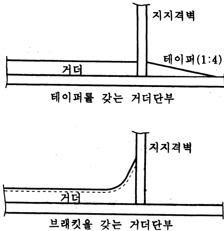
그림 3.5.11 거더의 단부
