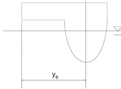
그림 3.2.1 쌍동선체의 y_b 정의
