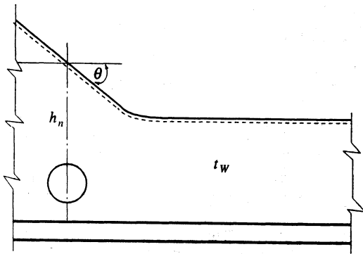
그림 3.5.14 브래킷주위의 유효 웨브 면적
