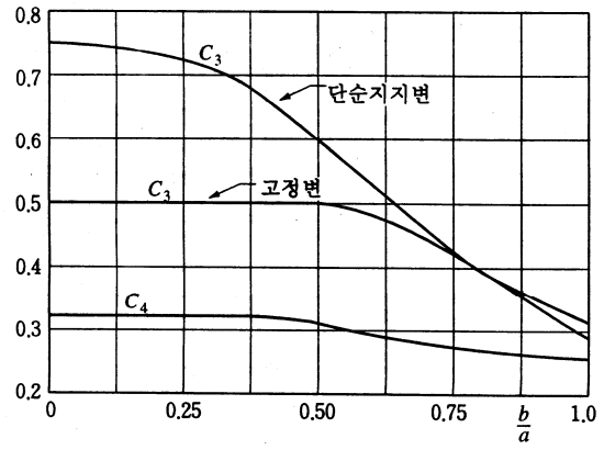
그림 3.5.10 계수 C_3 및 C_4
