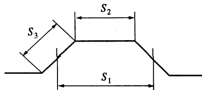
그림 3.3.1 파형격벽
