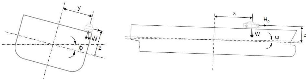
그림 1 선체운동
