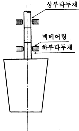
그림 4.4.1 스페이드 타(Spade rudder)
