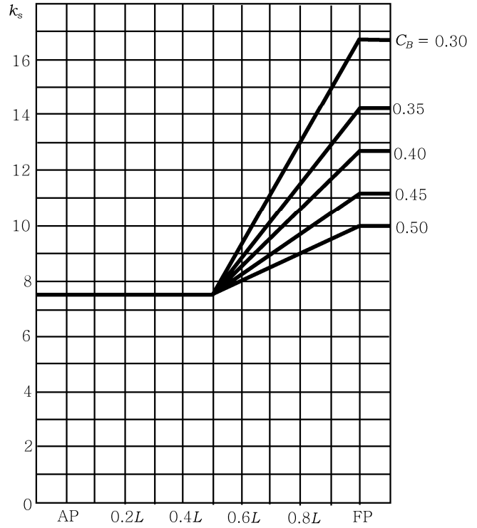
그림 3.2.8 해수압력 분포계수 k_s
