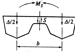
그림 3.2.12 횡방향 수직 굽힘모멘트 및 전단력
