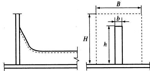
그림 3.5.15 유효접착면적
